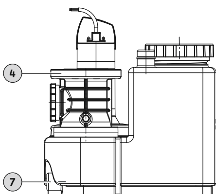
Fig. 7: Podłączanie ręcznej pompy membranowej
