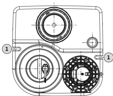
Fig. 2: Boven aanzicht opvoerinstallatie
