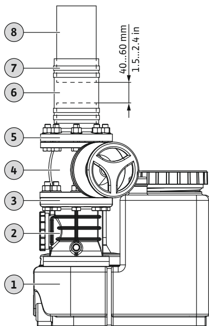
Fig. 3: Druckanschluss anbringen
