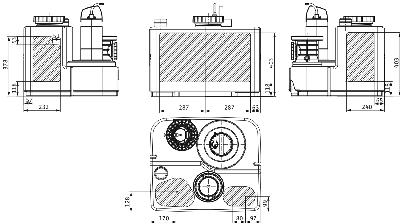
Fig. 4: Zulaufflächen
