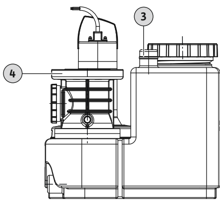
Fig. 6: Извод за обезвъздушаване на събирателния резервоар
