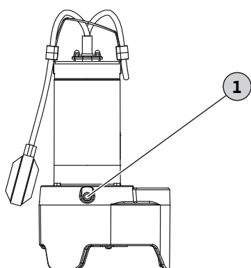
Fig. 3: Výmena oleja v tesniacej komore
