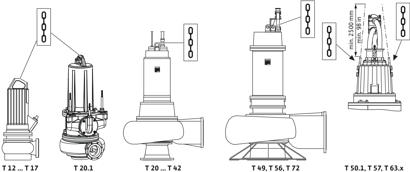
Fig. 2: Pritrdilne točke
