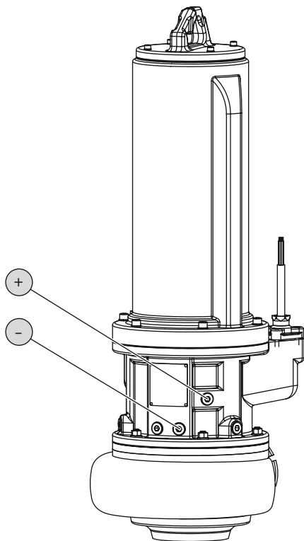
Fig. 5: Tätningsskammare: Kontrollera oljan
