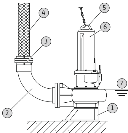
Fig. 7: Våt installation, bärbar
