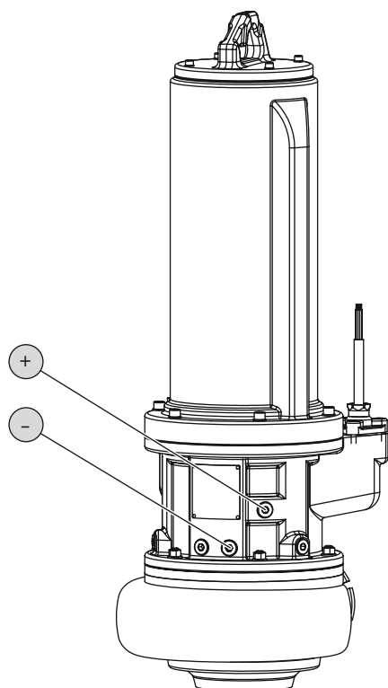
Fig. 11: Tätningskammare: Oljebyte
