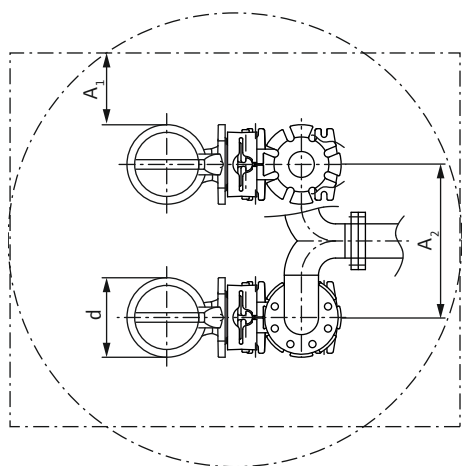
Fig. 3: Minsta avstånd
