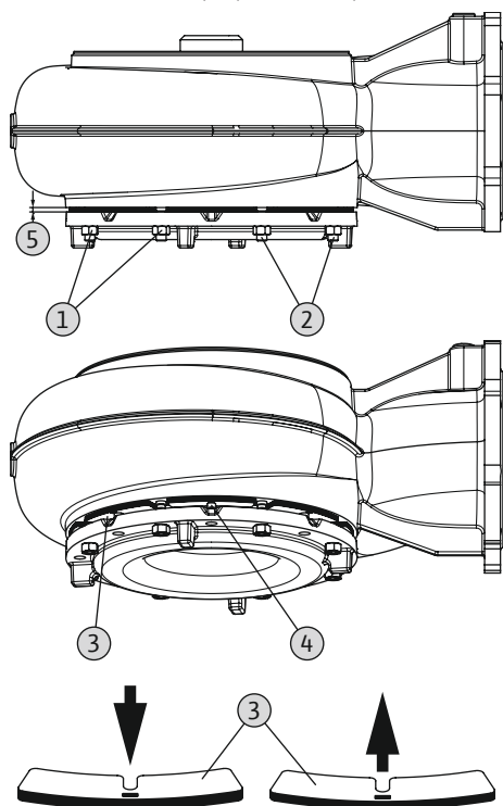
Fig. 13: SOLID G: Reglarea fantei
