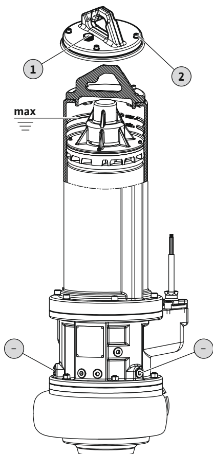
Fig. 4: Verificare agent de răcire
