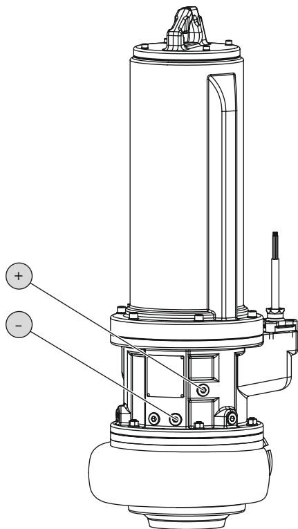
Fig. 5: Camera de etanșare: Verificarea uleiului
