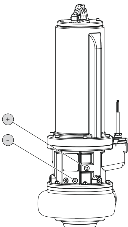
Fig. 11: Camera de etanșare: Schimb de ulei
