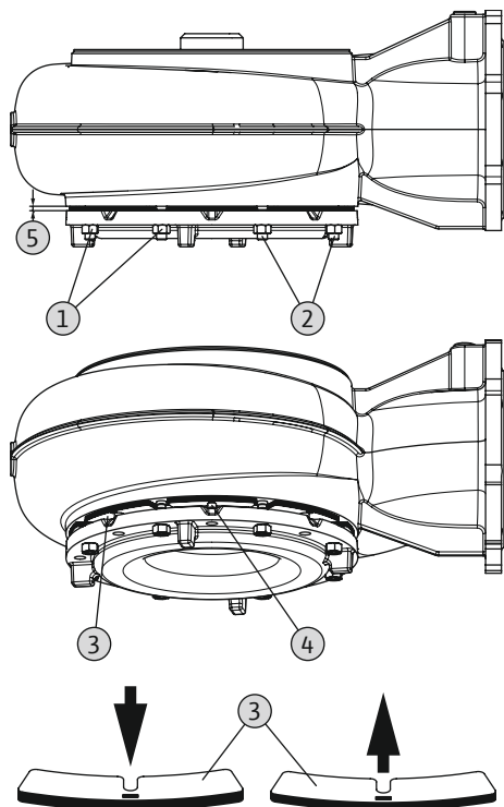
Fig. 13: SOLID G: Etterjustering av avstand
