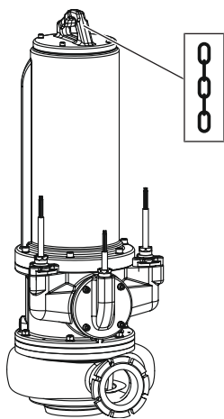
Fig. 2: Точка на подигнување
