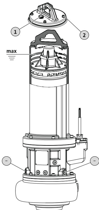
Fig. 4: Проверка на разладното средство
