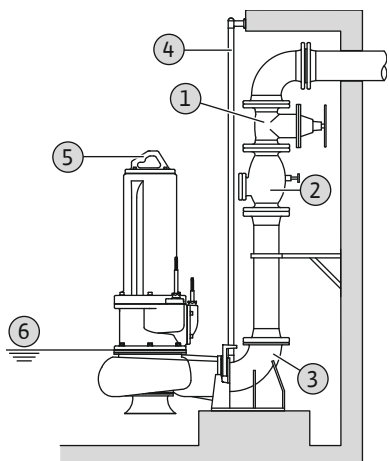
Fig. 6: Водено поставување, стационарно
