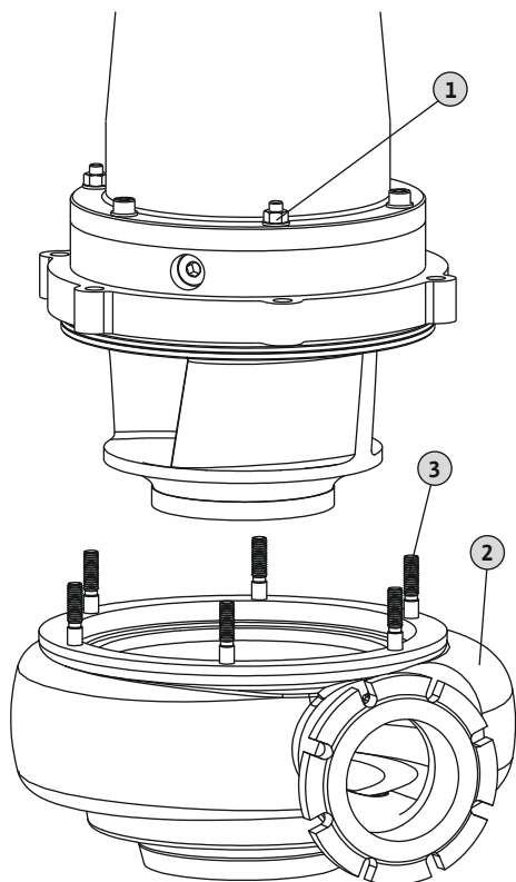
Fig. 12: Замена на хидрауличното куќиште
