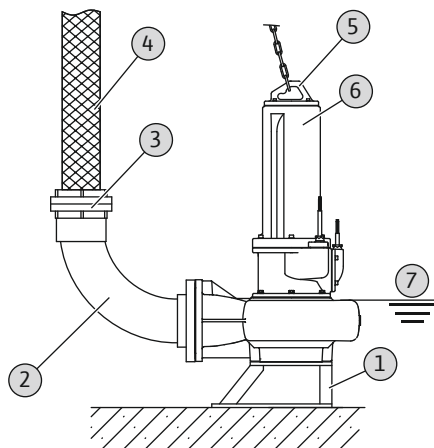
Fig. 7: Водено поставување, преносливо
