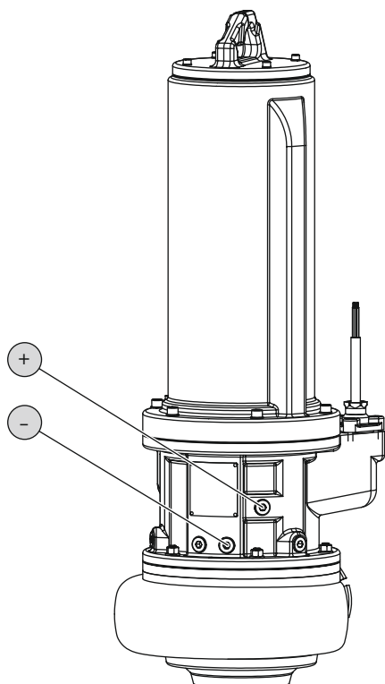
Fig. 11: Заптивна комора: Замена на масло
