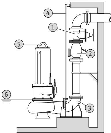
Fig. 6: Stacionārā uzstādīšana iegremdējot
