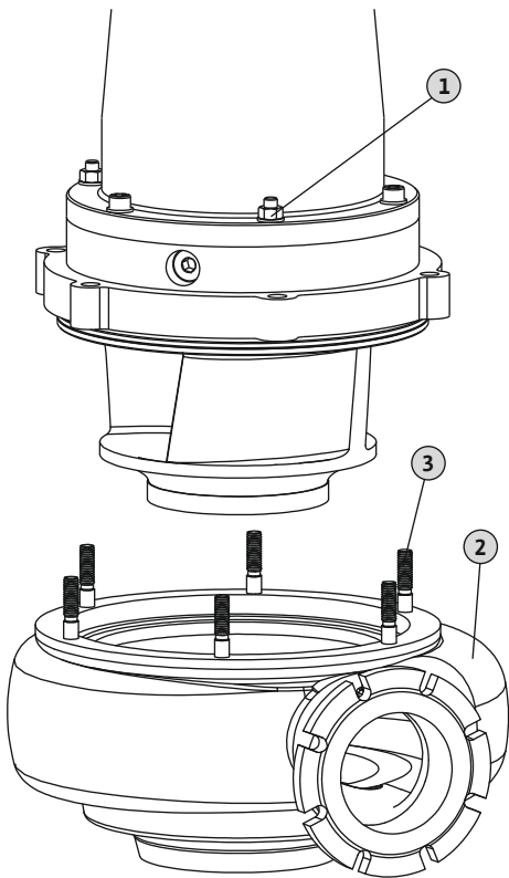
Fig. 12: Hidraulikas korpusa nomaiņa
