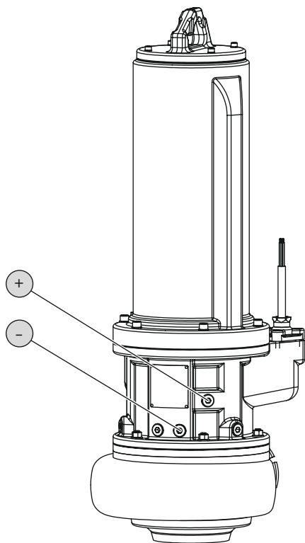
Fig. 5: Blīvēšanas kamera: Eļļas pārbaude
