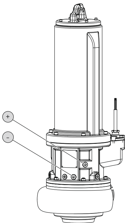
Fig. 11: Blīvēšanas kamera: Eļļas nomaīņa
