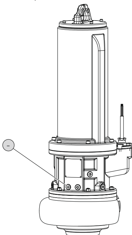
Fig. 9: Noplūdes kameras iztukšošana
