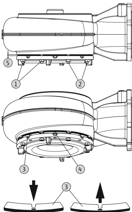
Fig. 13: SOLID G: atstarpes iestatīšana
