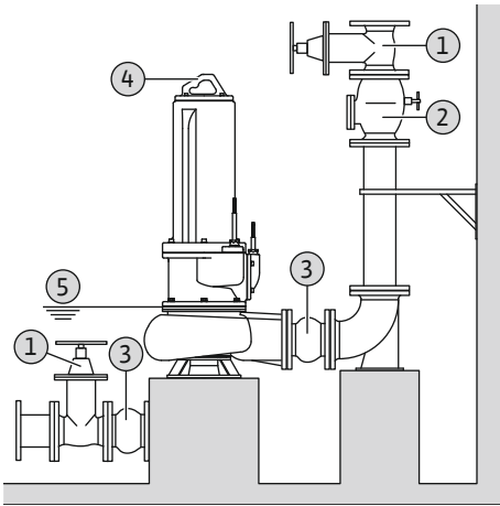
Fig. 8: Uztādīšana sausā vietā
