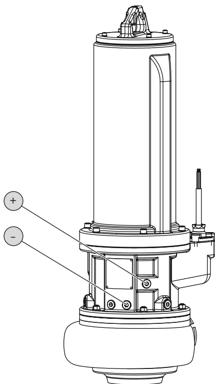
Fig. 11: Camera di tenuta: Cambio d'olio
