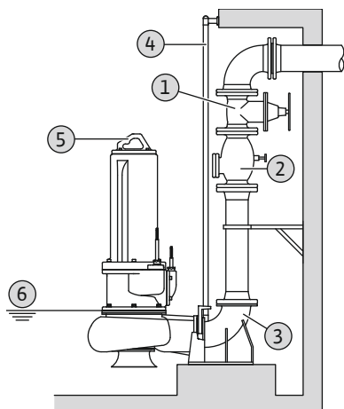
Fig. 6: Montaggio sommerso stazionario
