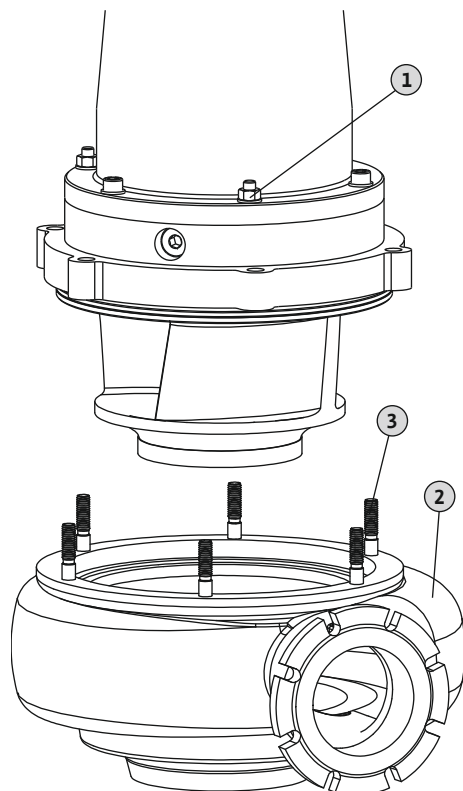
Fig. 12: Sostituire il corpo del gruppo idraulico
