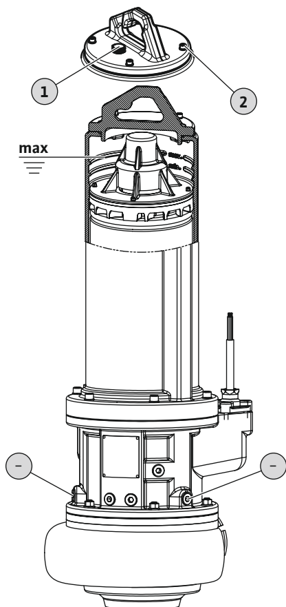
Fig. 4: Verificare il liquido di raffreddamento
