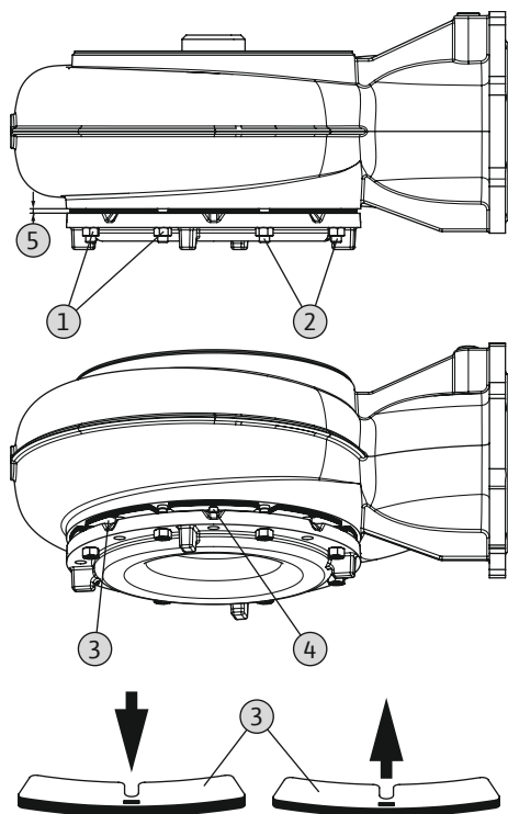
Fig. 13: SOLID G: A résméret utánállítása
