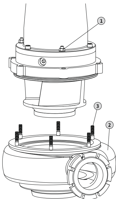
Fig. 12: A hidraulikaház cseréje
