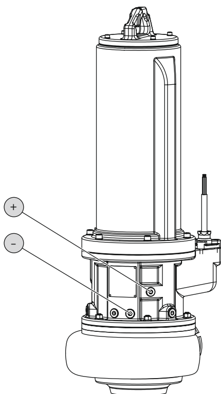
Fig. 11: Tömítőkamra: Olajcsere
