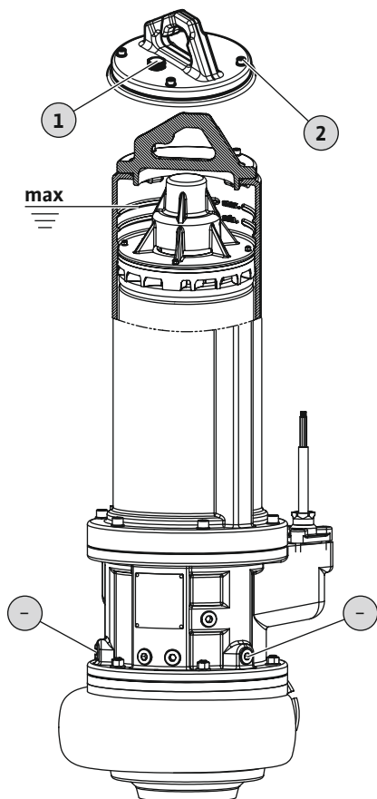
Fig. 4: A hűtőközeg ellenőrzése
