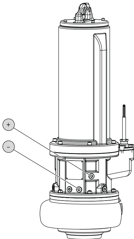
Fig. 5: Tömítőkamra: Az olaj ellenőrzése
