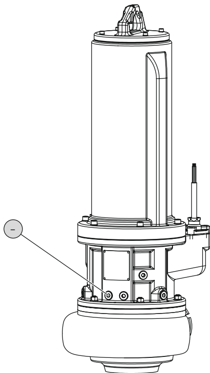
Fig. 9: Vidanger la chambre de fuite
