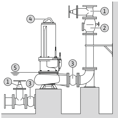
Fig. 8: Installation à sec
