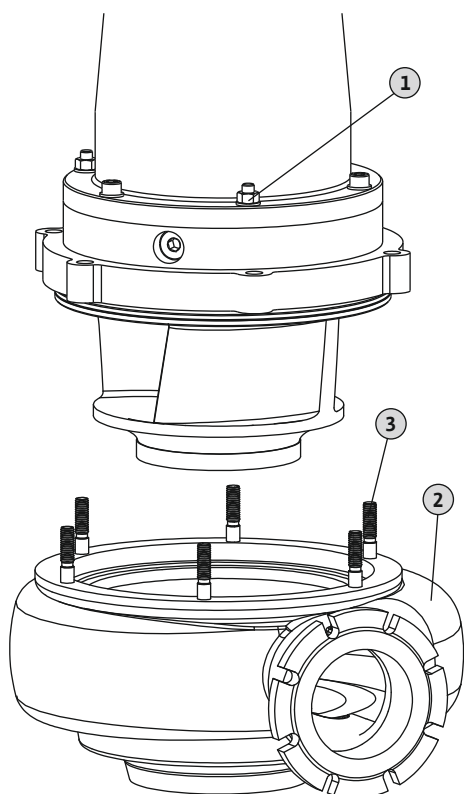
Fig. 12: Remplacement du corps hydraulique
