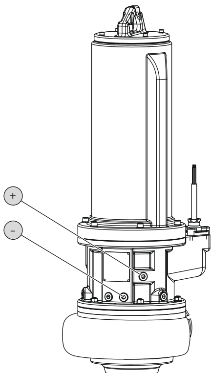
Fig. 11: Cámara de separación: Cambio de aceite
