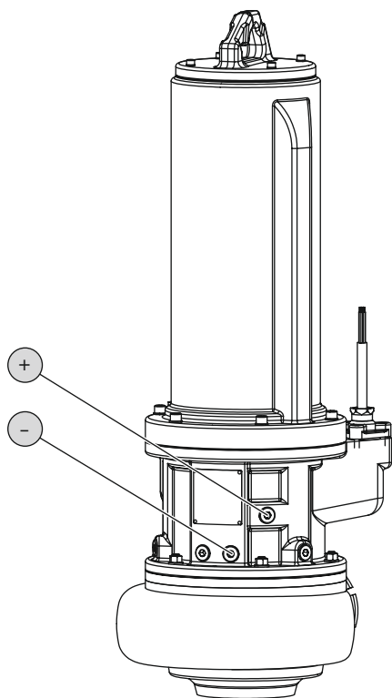
Fig. 5: Cámara de separación: Comprobar el aceite
