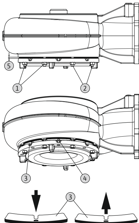
Fig. 13: SOLID G: Reajuste de la medida del espacio de separación
