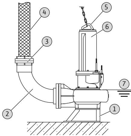
Fig. 7: Υγρή εγκατάσταση εντός φρεατίου, φορητή
