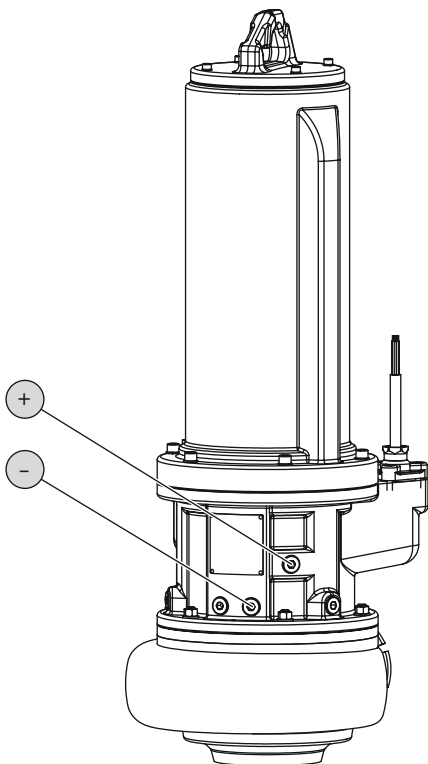
Fig. 11: Θάλαμος στεγανοποίησης: Αλλαγή λαδιού
