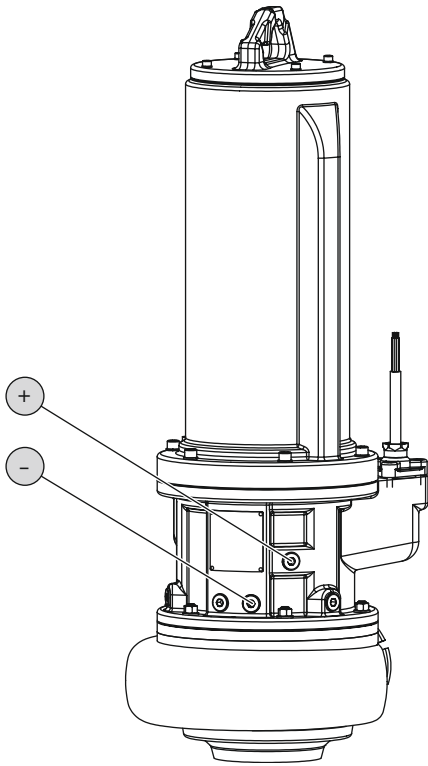
Fig. 5: Θάλαμος στεγανοποίησης: Έλεγχος του λαδιού
