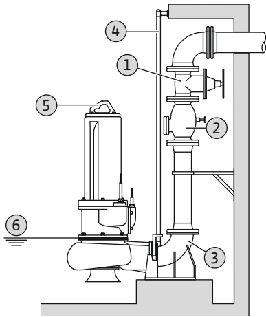
Fig. 6: Υγρή εγκατάσταση εντός φρεατίου, σταθερή
