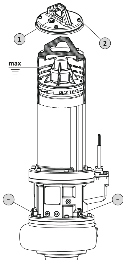
Fig. 4: Έλεγχος του ψυκτικού μέσου
