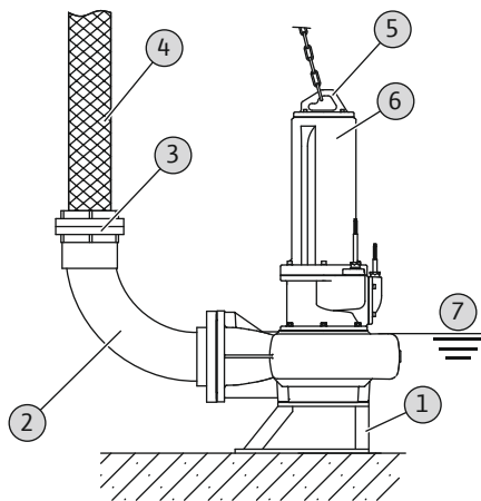
Fig. 7: Мокър монтаж, мобилен
