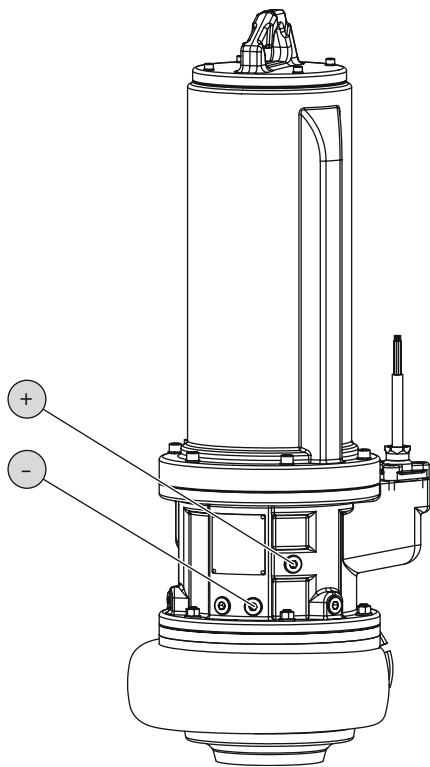
Fig. 5: Уплътнителна камера: Контролиране на маслото
