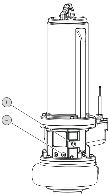
Fig. 11: Уплътнителна камера: Смяна на маслото
