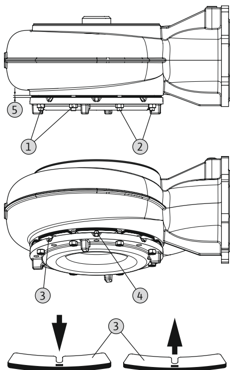
Fig. 13: SOLID G: Регулиране на размерите на разреза
