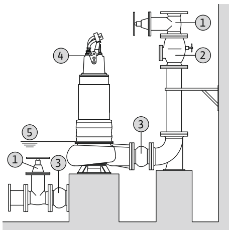
Fig. 12: Suchá inštalácia
