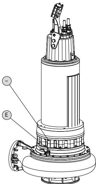
Fig. 16: Vypúšťanie presakovacej komory FKT 50.1, 57, 63.1
