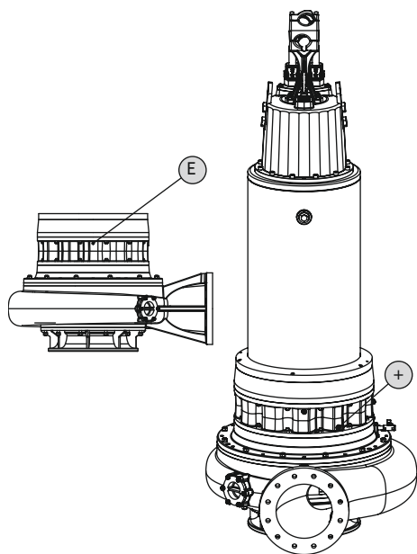
Fig. 20: Premazanie valivého ložiska FKT 50.1, 57, 63.1
