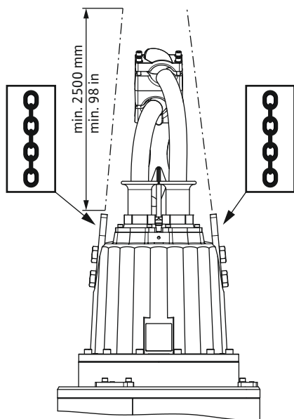
Fig. 2: Upevňovacie body
