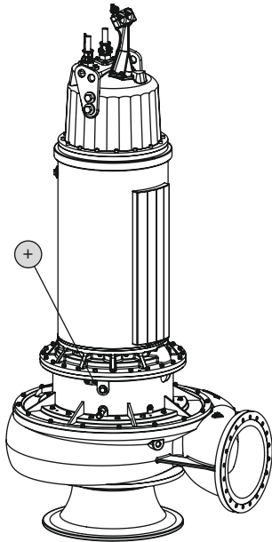
Fig. 21: Premazanie valivého ložiska FKT 63.2
