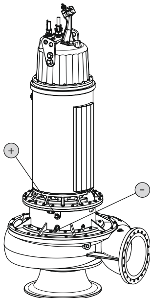
Fig. 10: Tesniaca komora: Kontrola oleja
