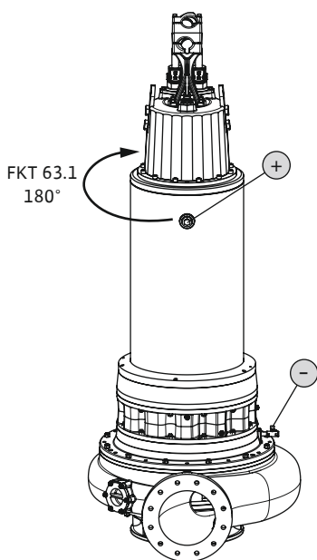
Fig. 14: Chladiaci systém: Výmena chladiaceho prostriedku FKT 50.1, 57, 63.1
