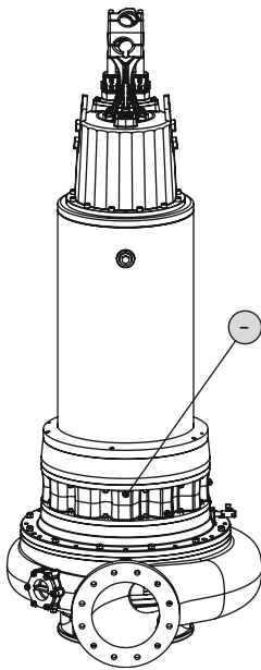
Fig. 18: Vypustenie kondenzovanej vody FKT 50.1, 57, 63.1
