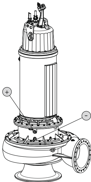
Fig. 10: Komora uszczelnienia: Sprawdzić poziom oleju
