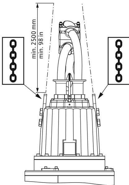
Fig. 2: Punkty mocowania
