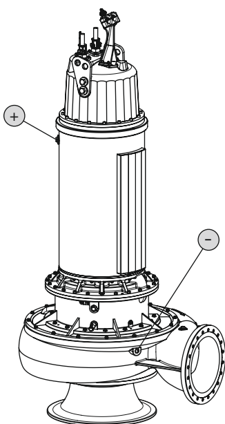
Fig. 9: Układ chłodzenia: Sprawdzić środek chłodzący FKT 63.2
