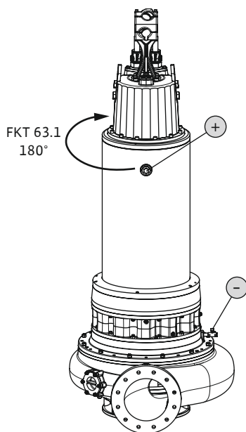
Fig. 8: Układ chłodzenia: Sprawdzić środek chłodzący FKT 50.1, 57, 63.1
