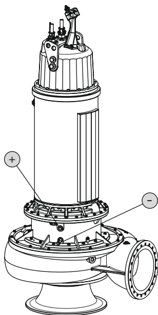
Fig. 13: Komora uszczelnienia: Wymiana oleju
