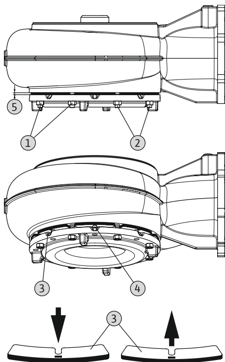
Fig. 23: SOLID G: Regulacja wymiaru szczeliny
