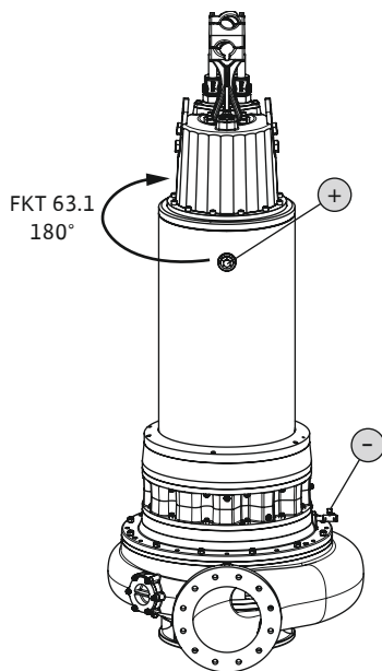
Fig. 14: Układ chłodzenia: Wymiana środka chłodzącego FKT 50.1, 57, 63.1
