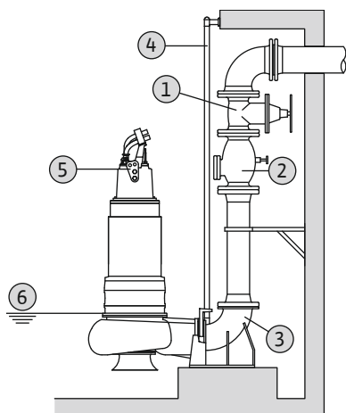
Fig. 11: Ustawienie mokre, stacjonarne
