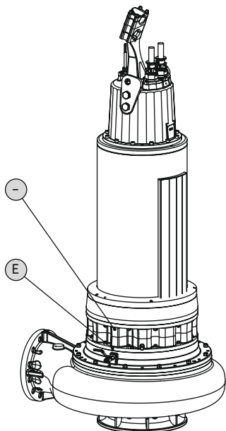
Fig. 16: Празнење на комора за протекување FKT 50.1, 57, 63.1
