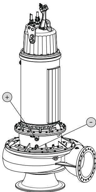
Fig. 13: Заптивна комора: Замена на масло
