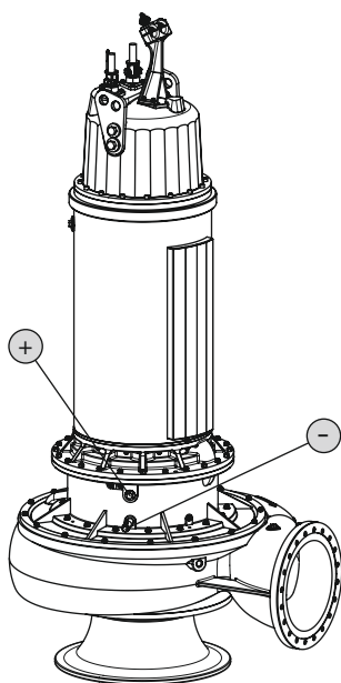
Fig. 10: Заптивна комора: Проверете го маслото
