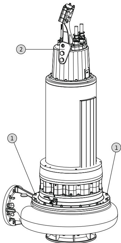
Fig. 22: Замена на хидраулично куќиште
