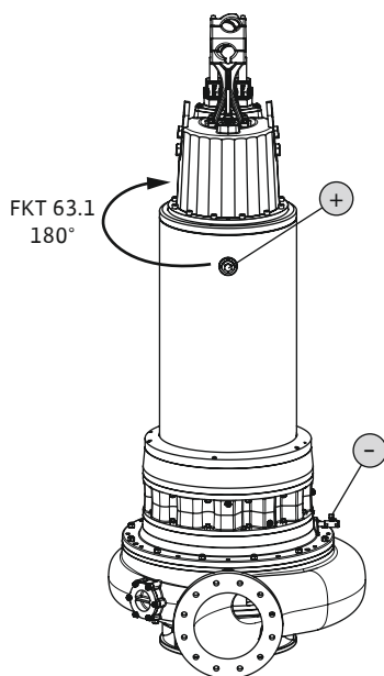
Fig. 8: Систем за ладење: Проверете го разладното средство FKT 50.1, 57, 63.1
