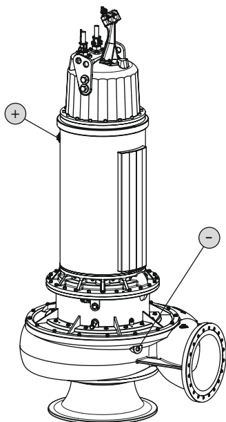
Fig. 15: Систем за ладење: Замена на разладно средство FKT 63.2
