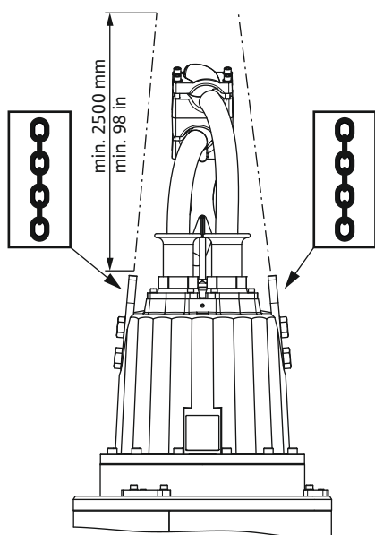
Fig. 2: Точки на подигнување
