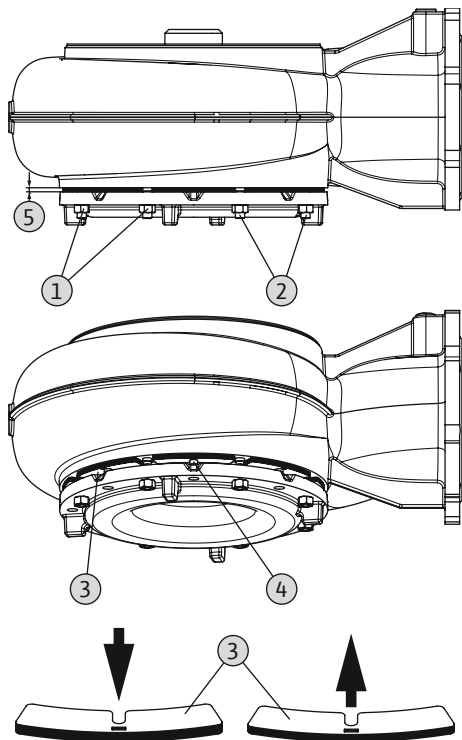
Fig. 23: SOLID G: Spleetmaat bijstellen
