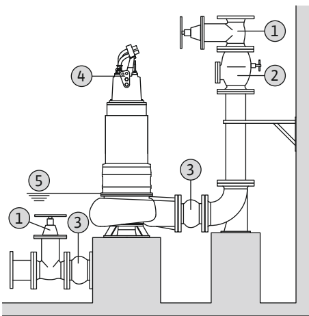
Fig. 12: Droge opstelling
