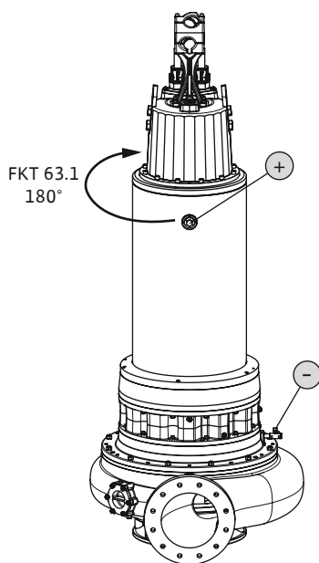
Fig. 14: Koelsysteem: Koelmiddel vervangen FKT 50.1, 57, 63.1
