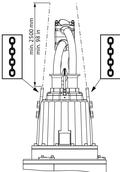
Fig. 2: Bevestigingspunten
