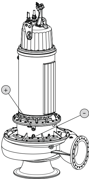
Fig. 10: Afdichtingsruimte: Oliepeil controleren
