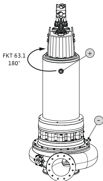
Fig. 8: Koelsysteem: Koelmiddel controleren FKT 50.1, 57, 63.1
