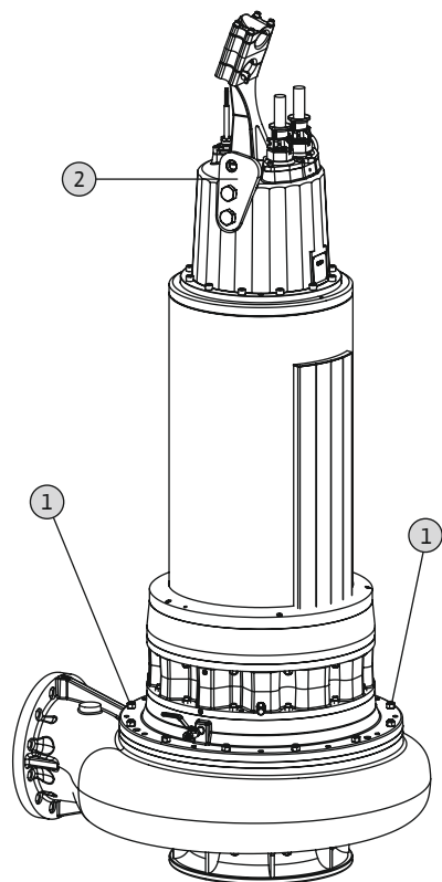
Fig. 22: Hydraulisch huis vervangen
