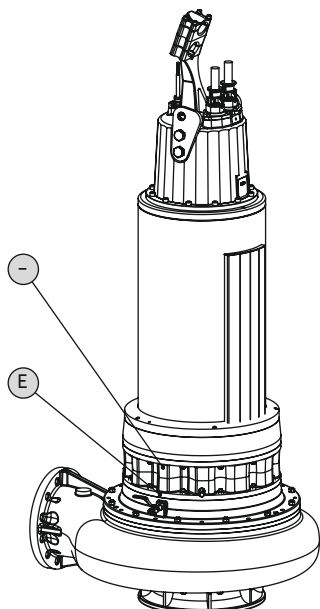
Fig. 16: Maak de lekkagekamer leeg FKT 50.1, 57, 63.1
