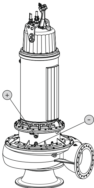
Fig. 13: Afdichtingsruimte: Olieverversen
