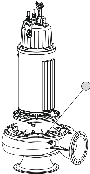
Fig. 17: Vuotokammion tyhjennys FKT 63.2
