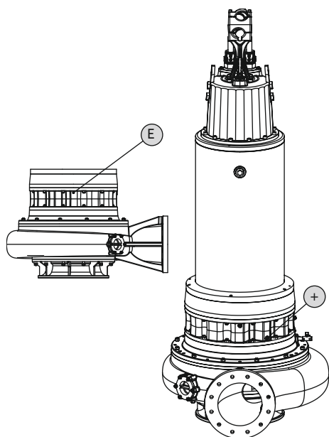
Fig. 20: Rullalaakerien jälkirasvaus FKT 50.1, 57, 63.1
