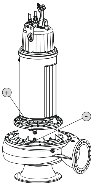
Fig. 13: Tiivistekammio: Öljyn vaihto
