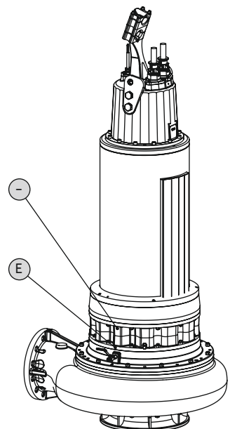
Fig. 16: Vuotokammion tyhjennys FKT 50.1, 57, 63.1
