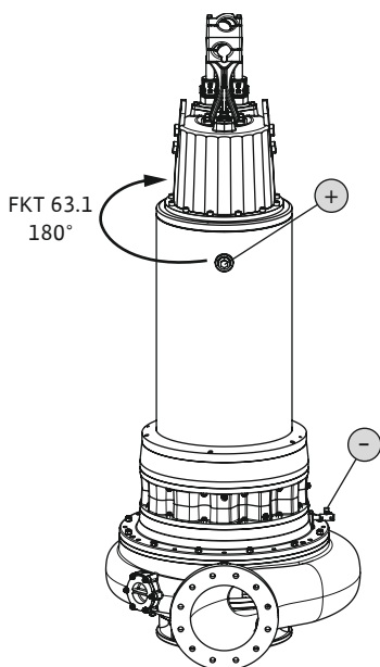
Fig. 14: Jäähdytysjärjestelmä: Jäähdytysnesteen vaihto FKT 50.1, 57, 63.1
