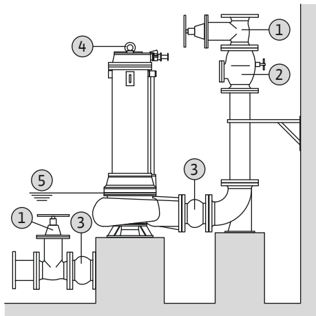
Fig. 10: Суха установка
