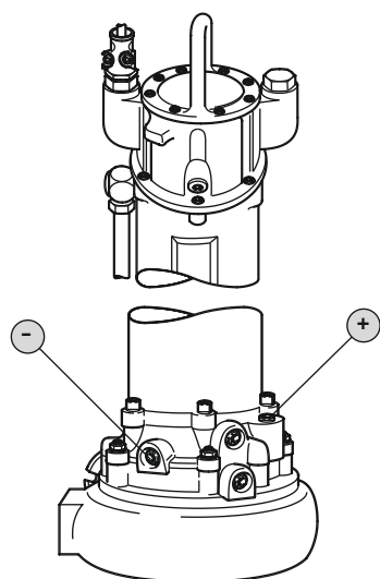
Fig. 14: Ущільнююча камера: Заміна мастила
