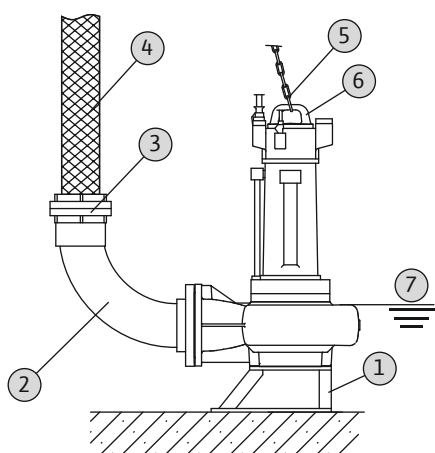
Fig. 9: Занурена установка, пересувна
