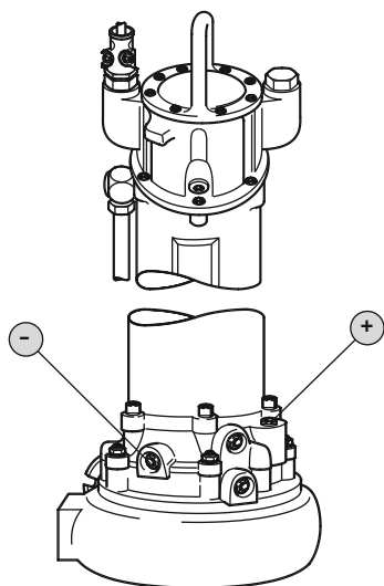
Fig. 7: Ущільнююча камера: перевірка мастила
