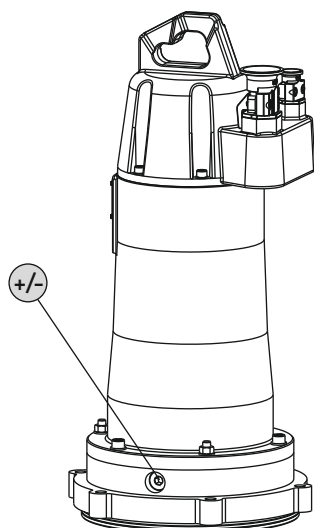
Fig. 13: Ущільнююча камера: Заміна мастила
