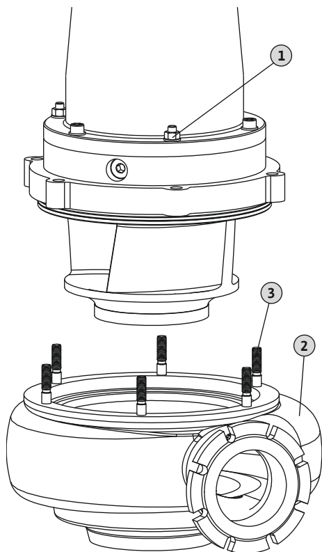
Fig. 15: Заміна корпусу гідравліки
