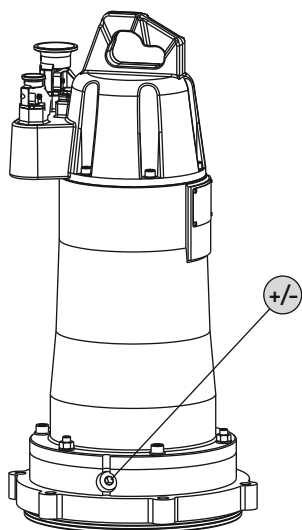
Fig. 4: Камера двигуна: перевірка мастила
