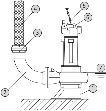
Fig. 9: Islak kurulum, taşınabilir
