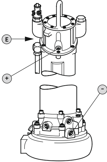
Fig. 12: Motor odası: Yağ değişimi
