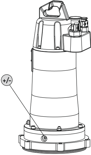
Fig. 6: Yalıtım haznesi: Yağın kontrol edilmesi
