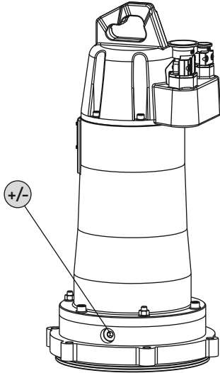
Fig. 13: Yalıtım haznesi: Yağ değişimi
