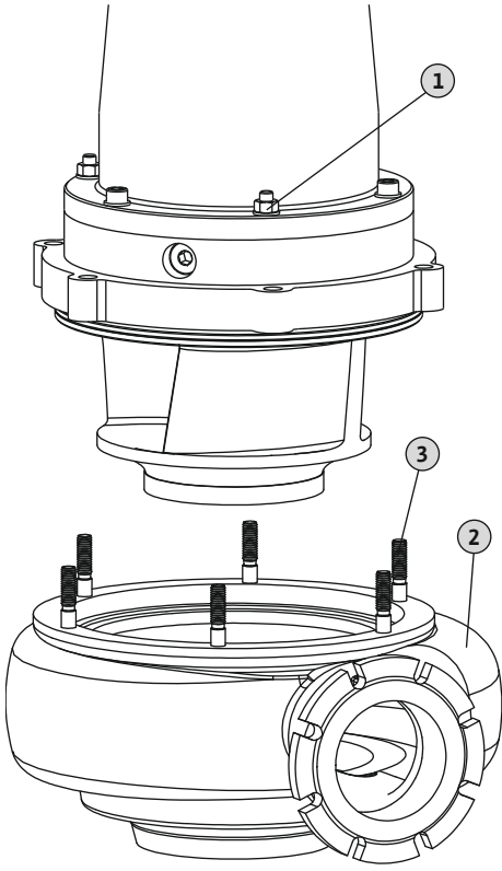
Fig. 15: Hidrolik gövdenin değiştirilmesi
