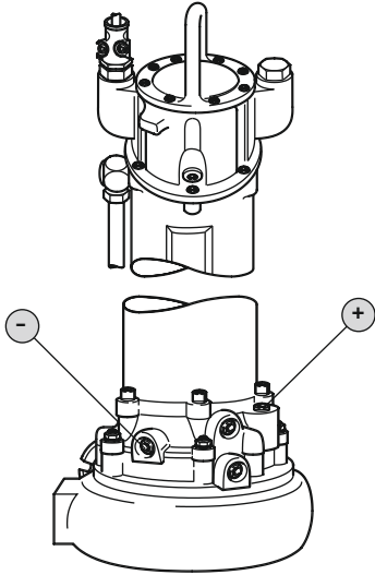
Fig. 7: Yalıtım haznesi: Yağın kontrol edilmesi
