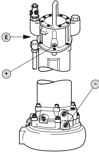
Fig. 5: Motor odası: Yağın kontrol edilmesi
