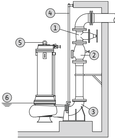
Fig. 8: Islak kurulum, sabit
