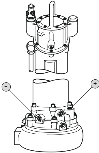
Fig. 14: Yalıtım haznesi: Yağ değişimi
