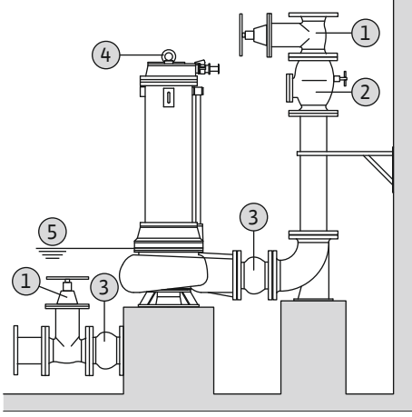
Fig. 10: Kuru kurulum
