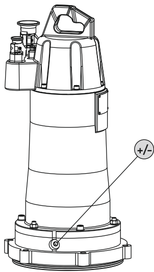
Fig. 11: Prostor za motor: Menjava olja
