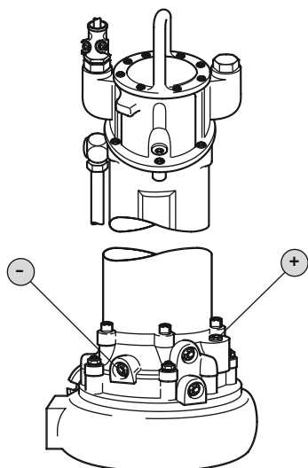
Fig. 7: Tesnilna komora: preverjanje olja
