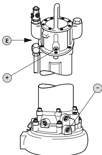
Fig. 5: Prostor za motor: preverjanje olja
