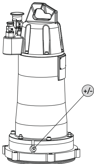
Fig. 4: Prostor za motor: preverjanje olja
