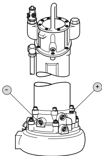
Fig. 14: Tesnilna komora: Menjava olja
