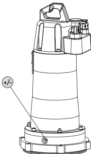
Fig. 13: Tesnilna komora: Menjava olja
