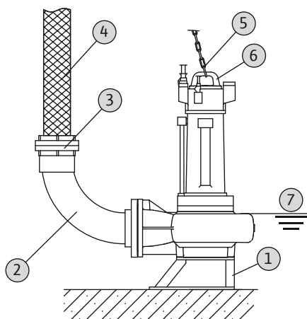
Fig. 9: Mokra montaža, prenosno
