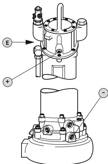
Fig. 5: Motorrum: Kontrol af olie
