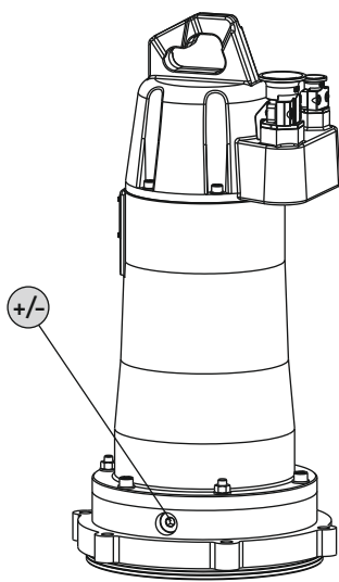
Fig. 13: Tætningskammer: Olieskift
