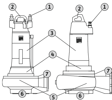
Fig. 1: Oversigt
