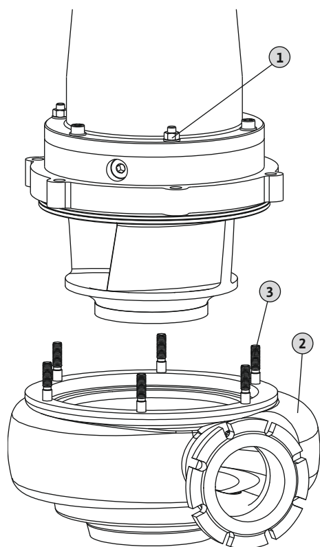
Fig. 15: Udskiftning af hydraulikhuset
