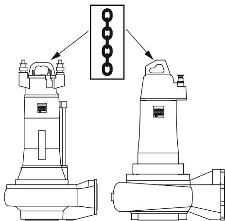
Fig. 2: Anhugningspunkt
