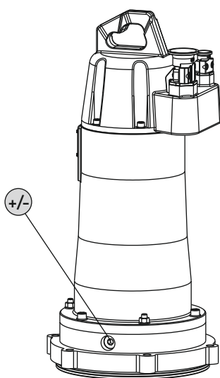
Fig. 6: Tætningskammer: Kontrol af olie
