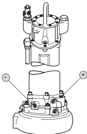
Fig. 14: Tætningskammer: Olieskift
