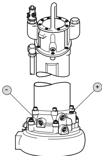
Fig. 7: Tætningskammer: Kontrol af olie
