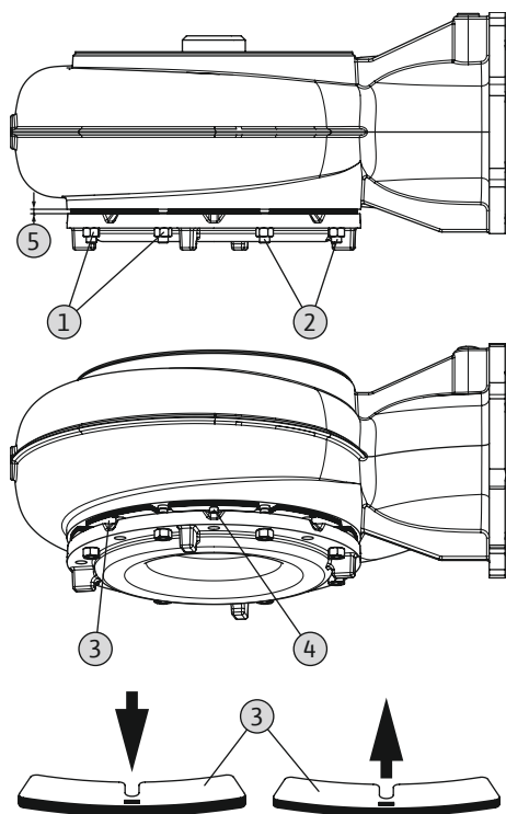
Fig. 16: SOLID G: Efterjustering af spaltemål
