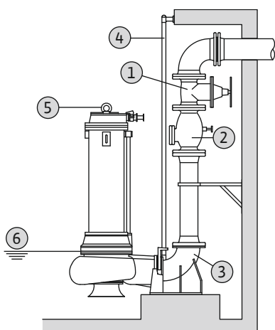
Fig. 8: Vådinstallation, stationær
