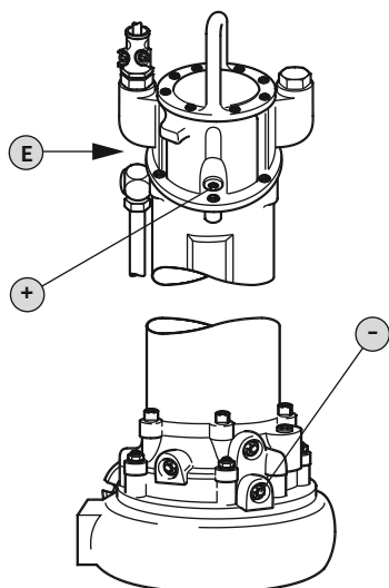
Fig. 12: Motorrum: Olieskift
