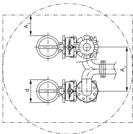
Fig. 3: Minimumafstande
