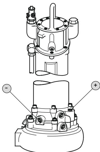
Fig. 14: Tetningskammer: Oljeskift
