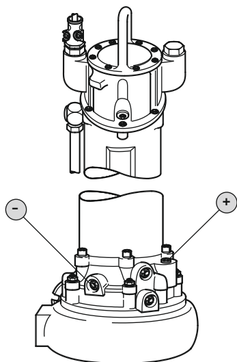
Fig. 7: Tetningskammer: Kontroller olje
