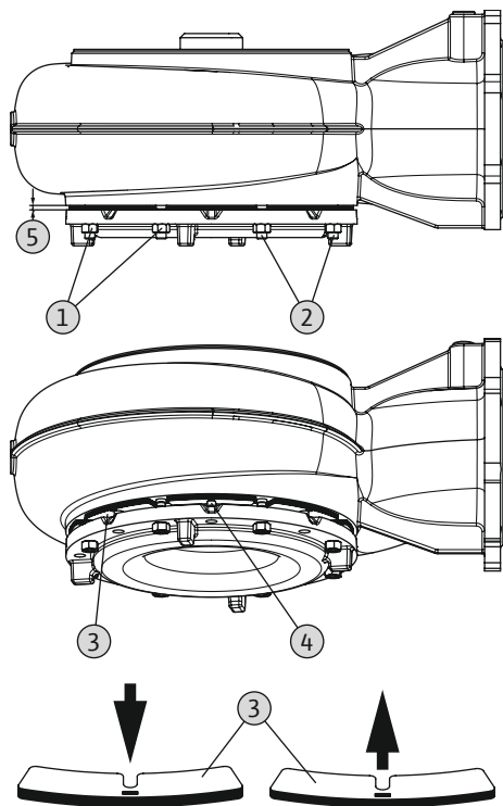
Fig. 16: SOLID G: Etterjustering av avstand
