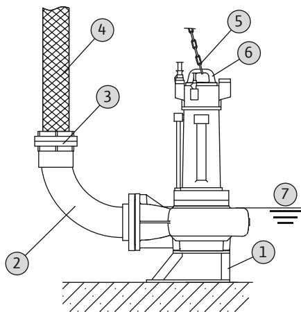
Fig. 9: Nedsenkbar installasjon, transportabel
