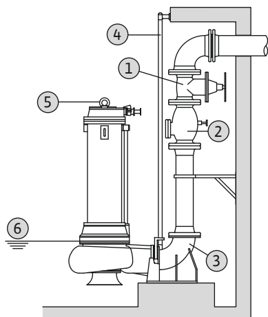
Fig. 8: Nedsenkbar installasjon, stasjonær
