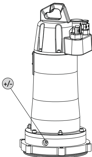
Fig. 6: Afdichtingsruimte: Olie controleren
