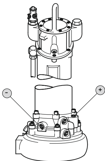
Fig. 7: Afdichtingsruimte: Olie controleren
