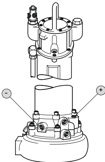
Fig. 14: Afdichtingsruimte: Olieverversen
