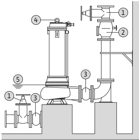
Fig. 10: Droge opstelling
