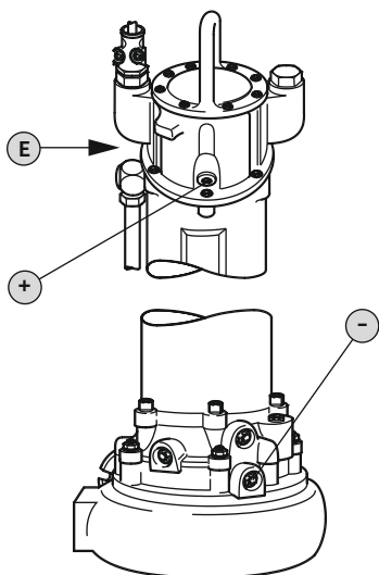
Fig. 5: Motorruimte: Olie controleren
