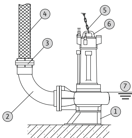
Fig. 9: Natte opstelling, mobiel
