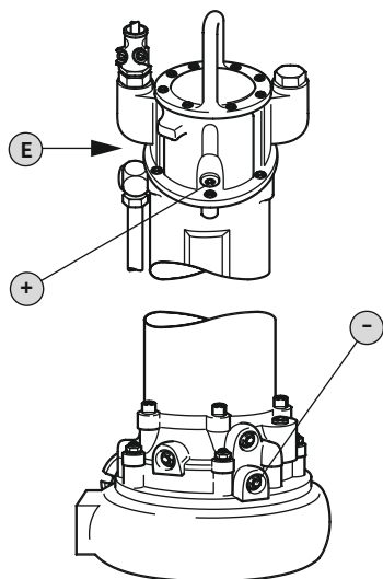
Fig. 12: Motorruimte: Olieverversen
