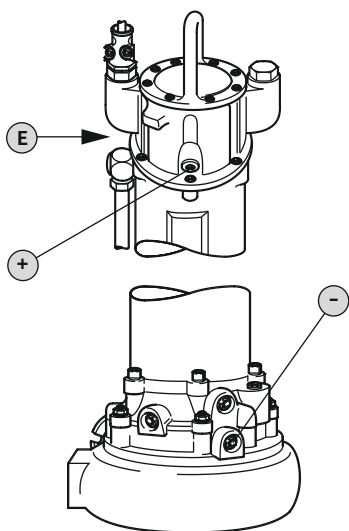
Fig. 5: Просторија на моторот: Проверете го маслото
