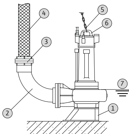
Fig. 9: Водено поставување, преносливо
