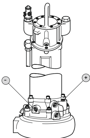
Fig. 14: Заптивна комора: Менување масло
