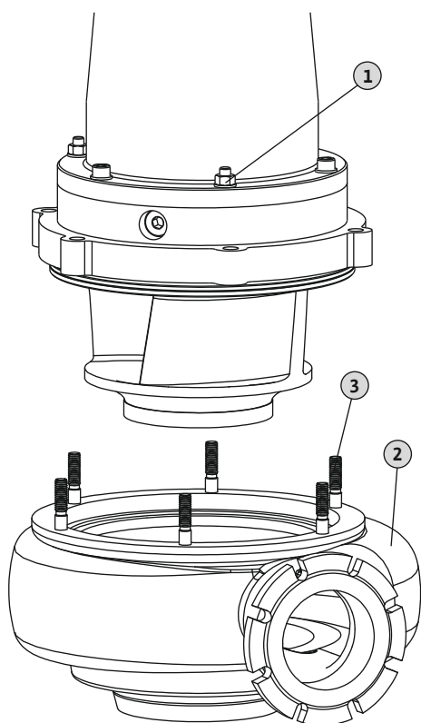
Fig. 15: Замена на хидрауличното куќиште
