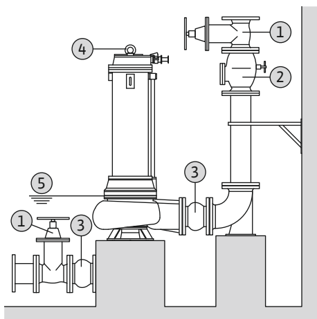
Fig. 10: Поставување на суво
