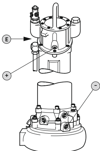
Fig. 12: Просторија на моторот: Менување масло
