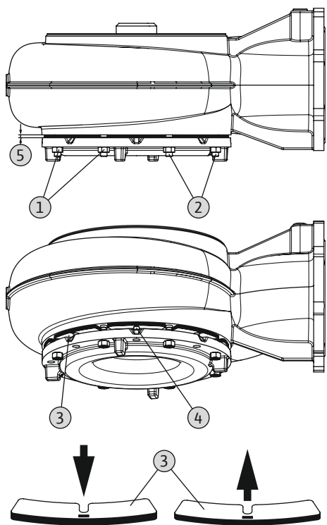
Fig. 16: SOLID G: Приспобување на празнината
