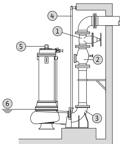
Fig. 8: Водено поставување, стационарно
