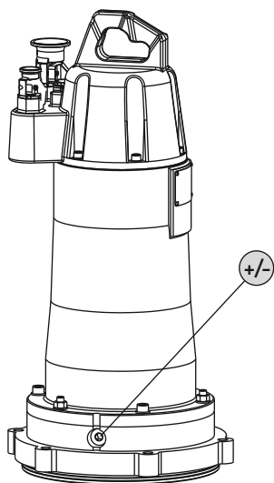
Fig. 4: Просторија на моторот: Проверете го маслото
