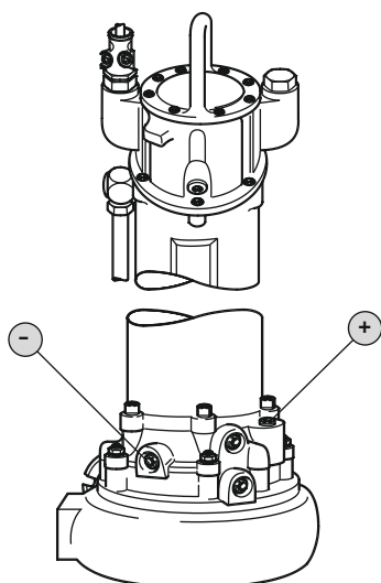
Fig. 7: Заптивна комора: Проверете го маслото
