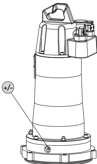
Fig. 13: Заптивна комора: Менување масло
