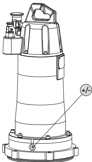
Fig. 11: Просторија на моторот: Менување масло
