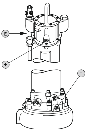
Fig. 12: Variklio skyrius: Alyvos pakeitimas
