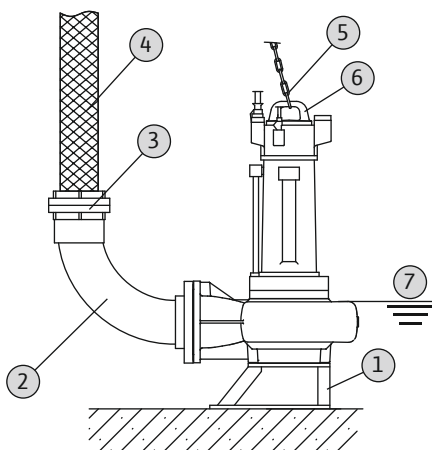
Fig. 9: Kilnojamas panardinamas montavimas
