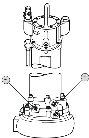
Fig. 7: Sandarinimo kamera: Patikrinkite alyvos lygį
