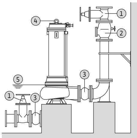
Fig. 10: Sausasis siurblių instaliavimas
