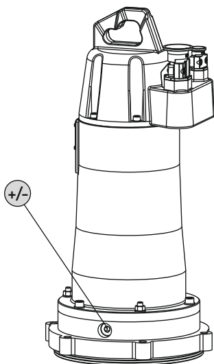
Fig. 6: Sandarinimo kamera: Patikrinkite alyvos lygį
