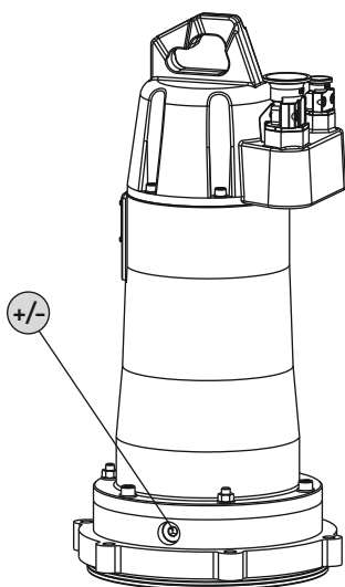
Fig. 13: Sandarinimo kamera: Alyvos pakeitimas
