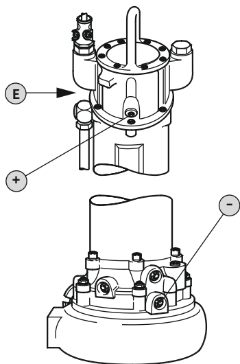
Fig. 5: Variklio skyrius: Patikrinkite alyvos lygį
