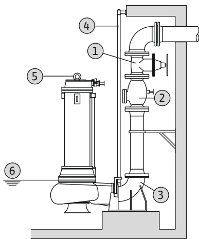
Fig. 8: Stacionarus panardinamas montavimas
