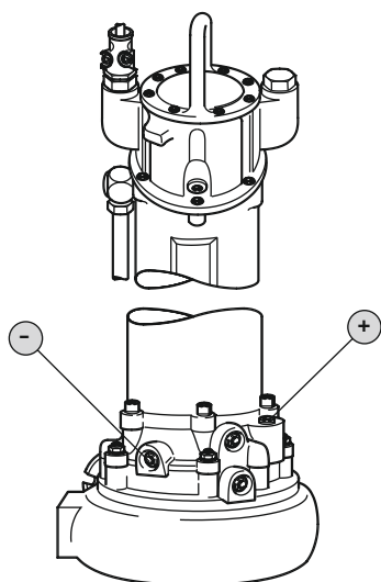
Fig. 7: Brtvena komora: Provjera razine ulja
