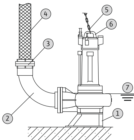
Fig. 9: Mokra ugradnja, prenosiva
