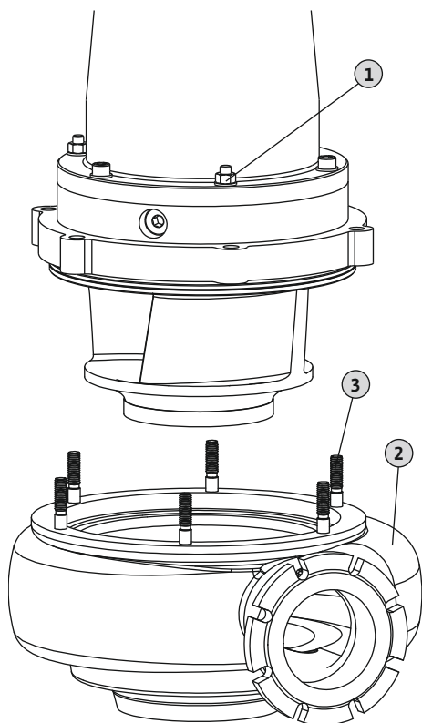
Fig. 15: Izmjena hidrauličkog kućišta
