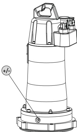
Fig. 6: Brtvena komora: Provjera razine ulja
