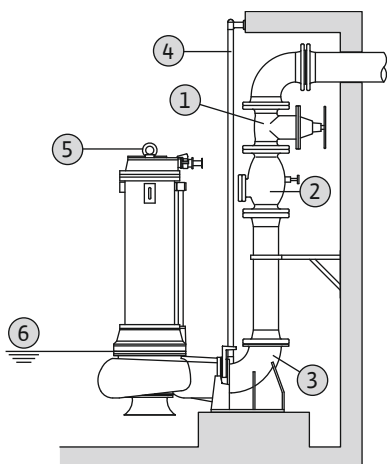
Fig. 8: Mokro postavljanje, stacionarno
