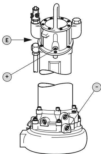
Fig. 12: Motorni prostor: Zamjena ulja
