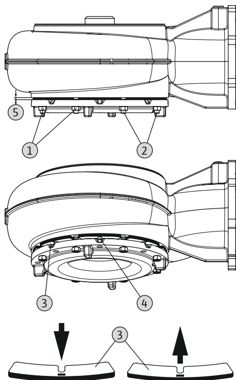
Fig. 16: SOLID G: Naknadno namještanje dimenzije razmaka
