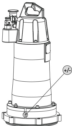
Fig. 4: Motorni prostor: Provjera razine ulja
