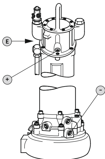
Fig. 5: Motorni prostor: Provjera razine ulja
