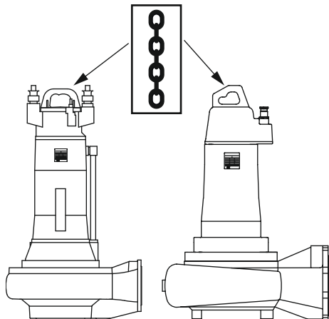
Fig. 2: Ovjesna točka
