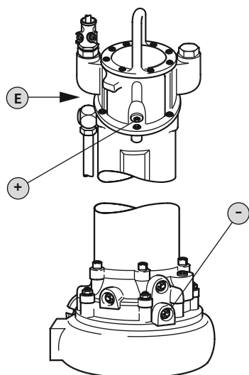
Fig. 12: Compartiment moteur : Vidange d'huile
