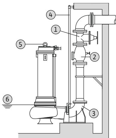
Fig. 8: Installation immergée stationnaire
