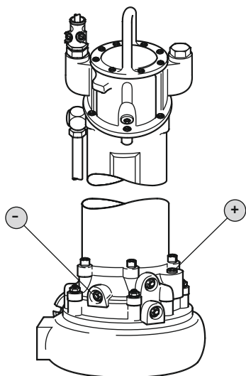
Fig. 14: Chambre d'étanchéité : Vidange d'huile
