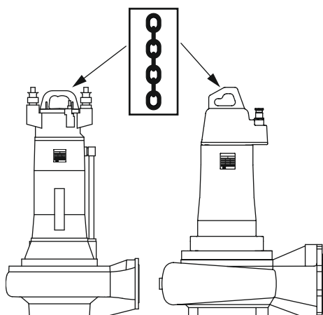
Fig. 2: Point d'élingage
