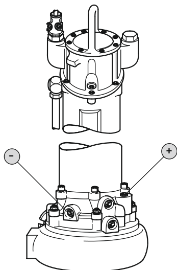
Fig. 14: Tiivistekammio: Öljyn vaihto
