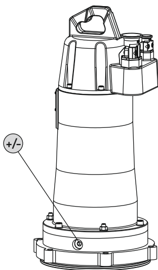
Fig. 6: Tiivistekammio: öljyn tarkistus
