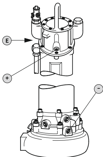
Fig. 5: Moottoritila: öljyn tarkistus
