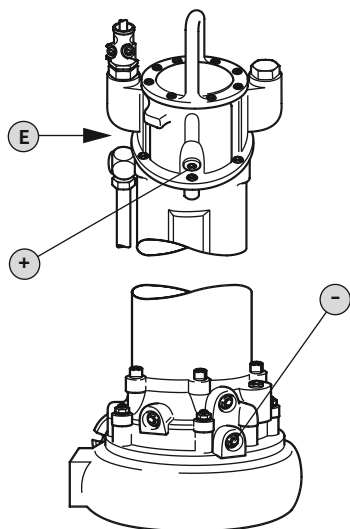
Fig. 12: Moottoritila: Öljyn vaihto
