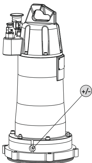
Fig. 4: Moottoritila: öljyn tarkistus
