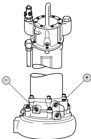
Fig. 7: Tiivistekammio: öljyn tarkistus
