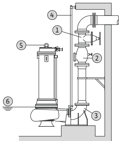
Fig. 8: Statsionaarne märgpaigaldus
