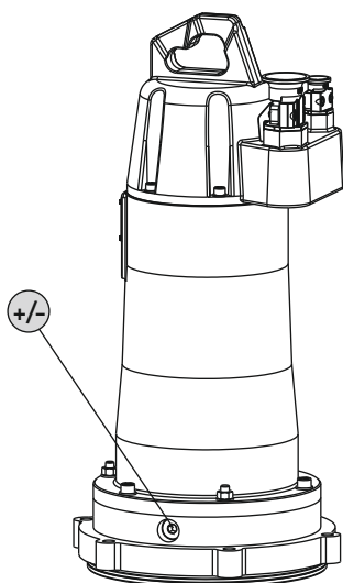
Fig. 6: Tihenduskamber: õli kontrollimine
