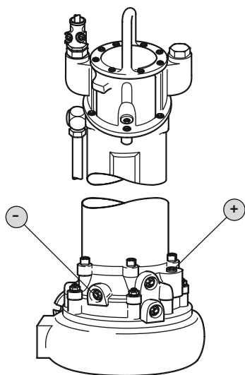
Fig. 14: Tihenduskamber: Õlivahetus
