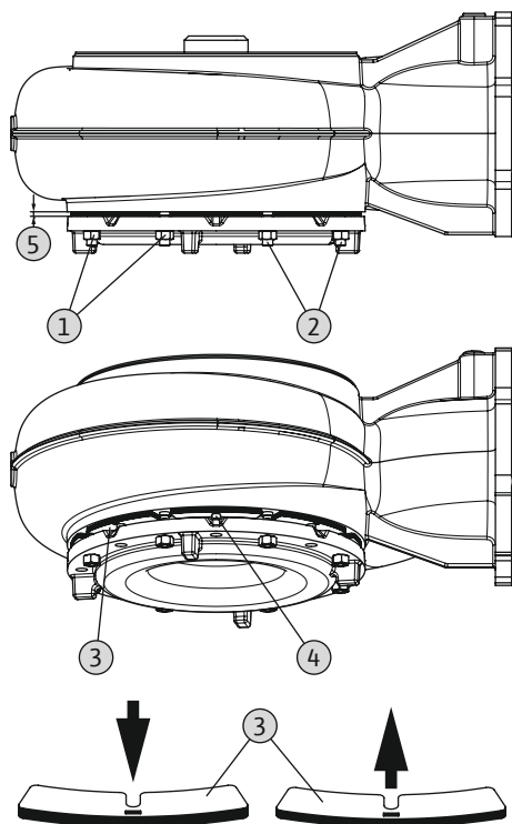
Fig. 16: SOLID G: Vahemaa reguleerimine
