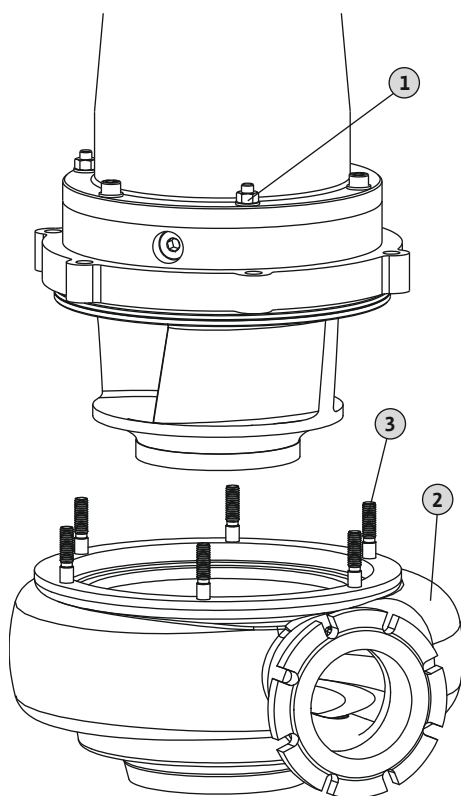
Fig. 15: Hüdraulikakorpuse vahetamine
