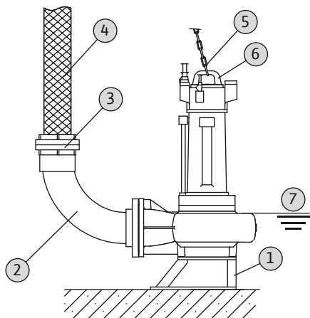
Fig. 9: Transporditav märgpaigaldus
