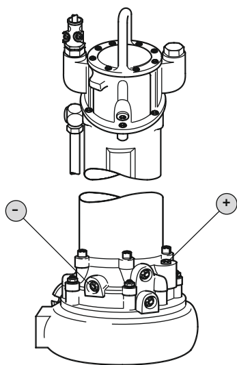
Fig. 7: Tihenduskamber: õli kontrollimine
