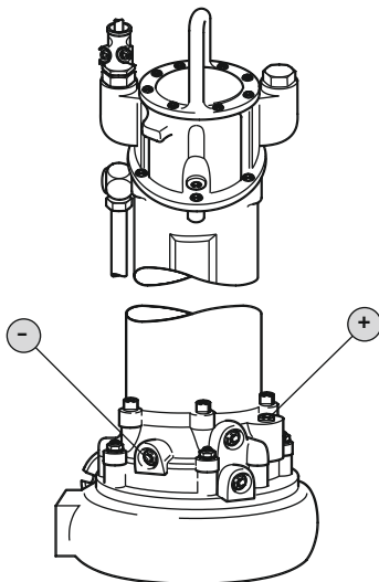
Fig. 7: Θάλαμος στεγανοποίησης: Έλεγχος του λαδιού
