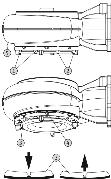
Fig. 16: SOLID G: Ρύθμιση κενού
