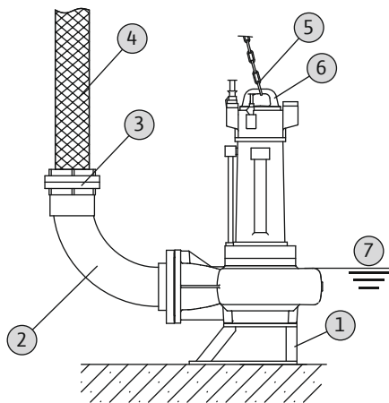
Fig. 9: Υγρή εγκατάσταση εντός φρεατίου, φορητή
