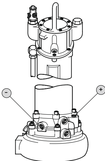
Fig. 14: Θάλαμος στεγανοποίησης: Αλλαγή λαδιού
