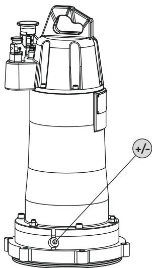
Fig. 11: Χώρος κινητήρα: Αλλαγή λαδιού
