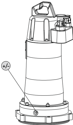
Fig. 6: Θάλαμος στεγανοποίησης: Έλεγχος του λαδιού
