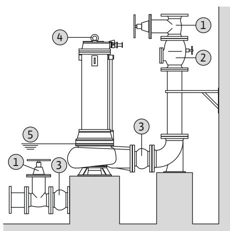
Fig. 10: Εγκατάσταση ξηρής τοποθέτησης
