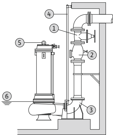
Fig. 8: Υγρή εγκατάσταση εντός φρεατίου, σταθερή
