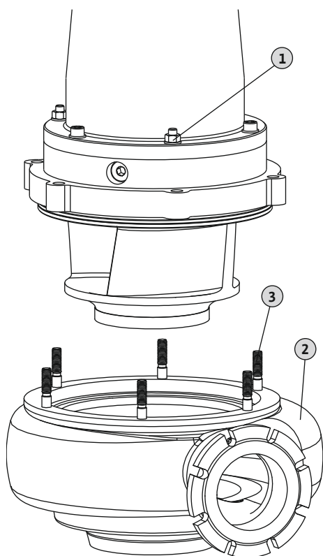
Fig. 15: Αντικατάσταση περιβλήματος υδραυλικού τμήματος
