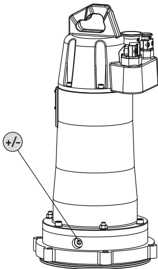
Fig. 13: Θάλαμος στεγανοποίησης: Αλλαγή λαδιού
