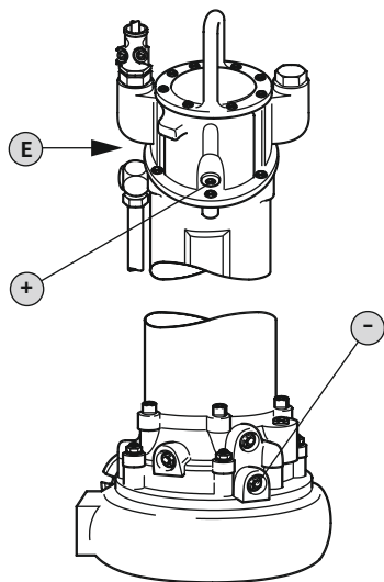
Fig. 5: Помещение на електродвигателя: Контролиране на маслото
