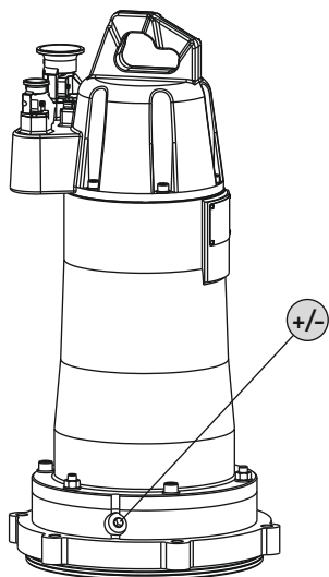
Fig. 11: Помещение на електродвигателя: Смяна на маслото
