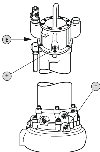
Fig. 12: Помещение на електродвигателя: Смяна на маслото
