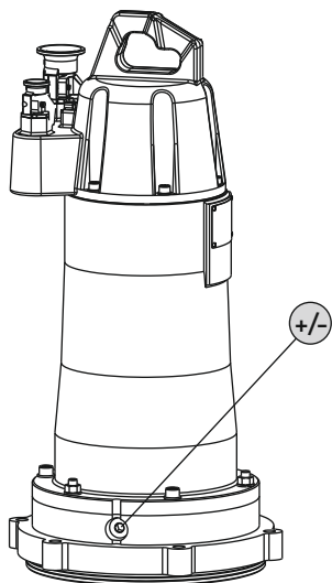
Fig. 4: Помещение на електродвигателя: Контролиране на маслото
