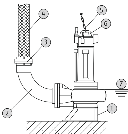
Fig. 9: Мокър монтаж, мобилен
