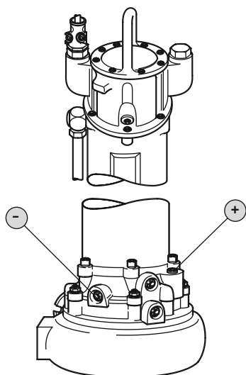
Fig. 7: Уплътнителна камера: Контролиране на маслото
