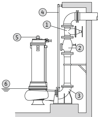
Fig. 8: Мокър монтаж, стационарен
