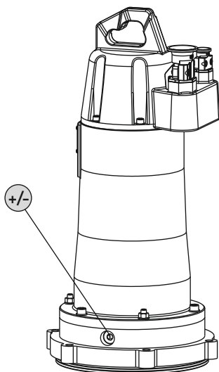
Fig. 6: Уплътнителна камера: Контролиране на маслото
