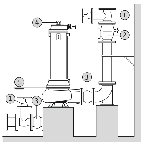
Fig. 10: Сух монтаж
