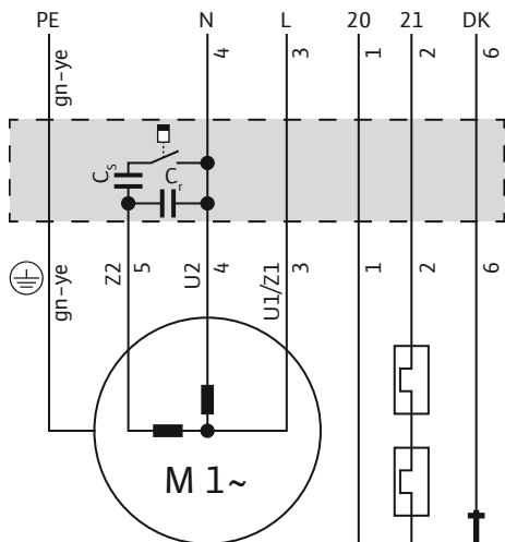
Fig. 7: Kablingsskjema vekselstrømsmotor
