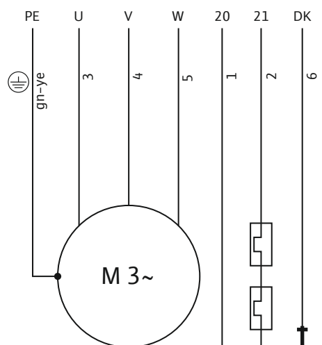
Fig. 8: Kablingsskjema: Direktestart, bimettalføler
