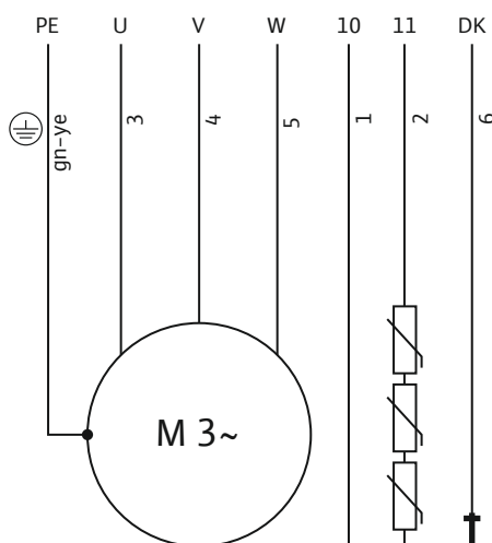
Fig. 9: Koblingskjema: Direktestart, PTC-sensor
