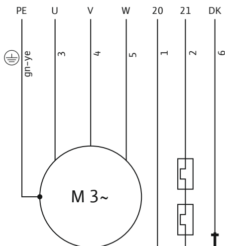
Fig. 8: Schema degli allacciamenti: Avviamento diretto, sensore bimetallo
