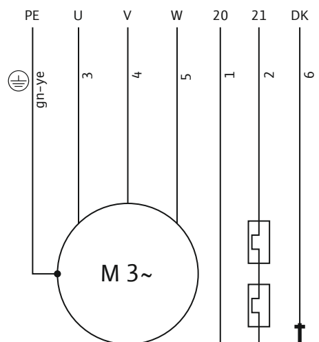
Fig. 8: Схема на свързване: Директно свързване, биметален сензор
