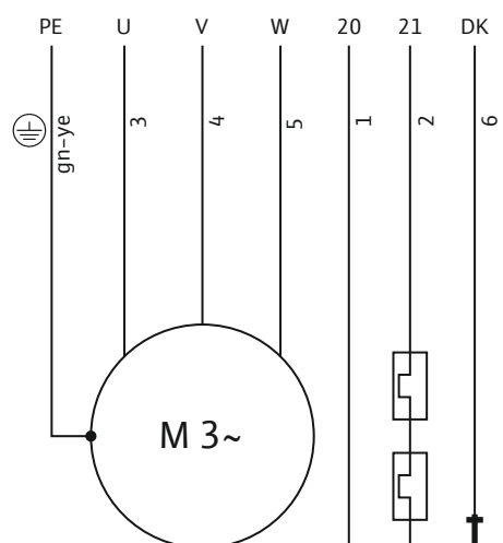
Fig. 8: Tilslutningsdiagram: Direkte start, bime-talføler
