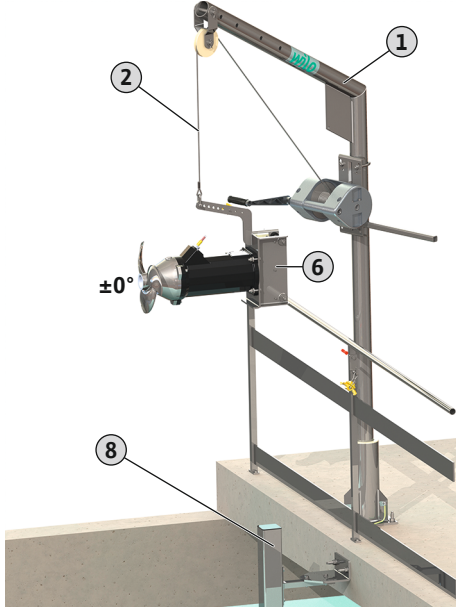
Fig. 6: Karıştırma düzenini havuzun üzerine döndürün
