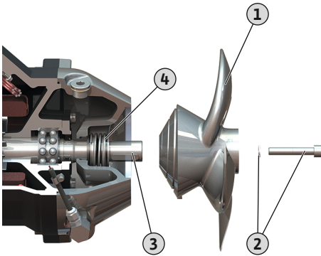
Fig. 13: Pervane değişimi
