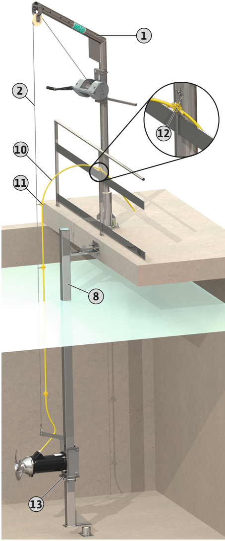
Fig. 8: Karıştırma düzeni, sabit dayanağa indirildi
