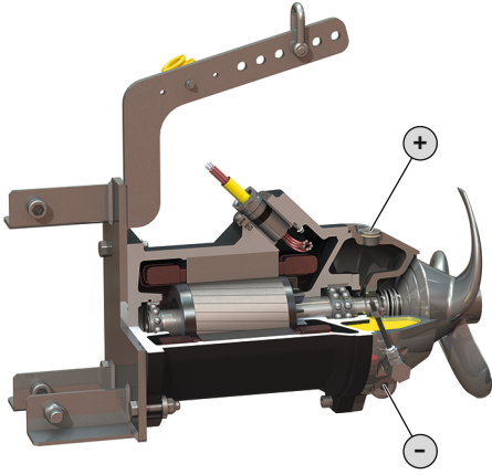
Fig. 12: Yağ değişimi
