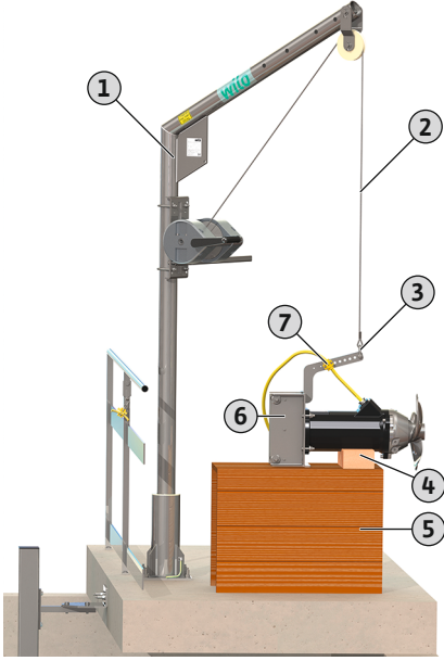
Fig. 5: Karıştırma düzenini hazırlama
