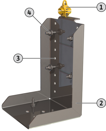
Fig. 16: Tabana montaj için konsol
