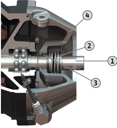
Fig. 14: Mekanik salmastra değişimi
