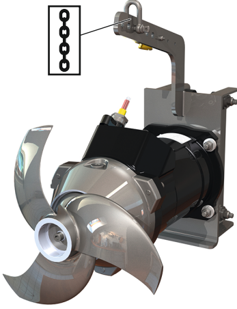
Fig. 1: Bağlama noktası
