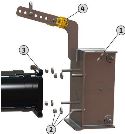
Fig. 15: Çerçeveyi değiştirme
