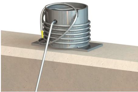
Fig. 9: Kaldırma aracı halat babasında emniyete alındı
