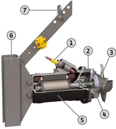
Fig. 2: Dalgıç motorlu karıştırma düzeneğine genel bakış
