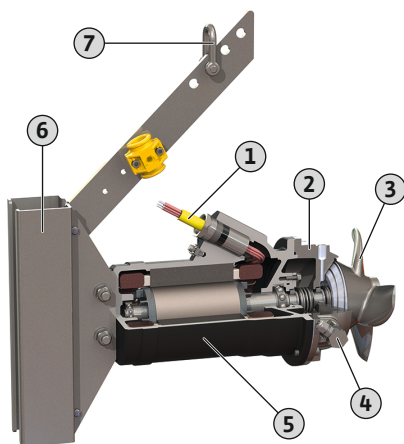
Fig. 2: Преглед на мешалката со потопен мотор
