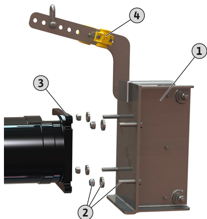
Fig. 15: Замена на рамка
