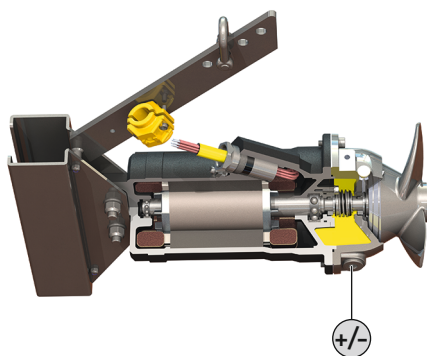
Fig. 11: Менување масло
