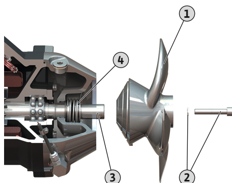
Fig. 13: Замена на пропелер
