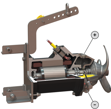
Fig. 12: Менување масло
