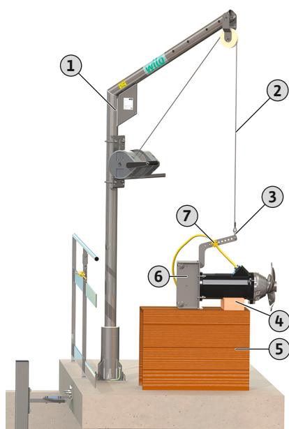
Fig. 5: Подготвување на погонот за мешање
