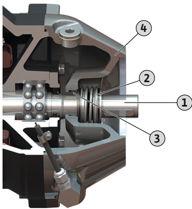
Fig. 14: Mechaninio sandariklio pakeitimas
