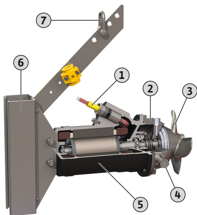
Fig. 2: Panardinamojo variklio maišytuvo apžvalga
