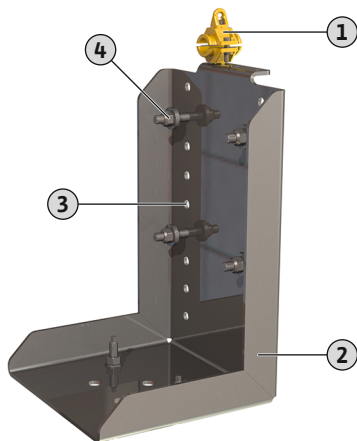
Fig. 16: Gembė tvirtinimui ant pagrindo
