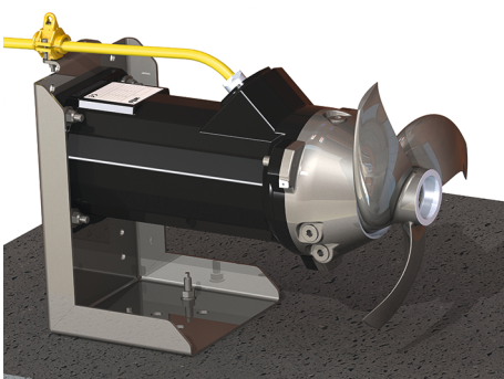
Fig. 4: Επιδαπέδια εγκατάσταση
