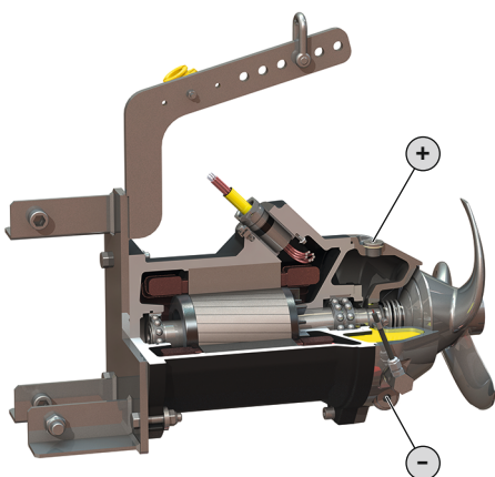
Fig. 12: Αλλαγή λαδιού
