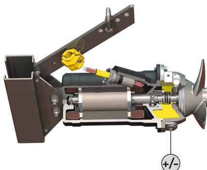
Fig. 11: Αλλαγή λαδιού
