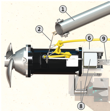
Fig. 7: Αναδευτήρας στη διάταξη καθέλκυσης
