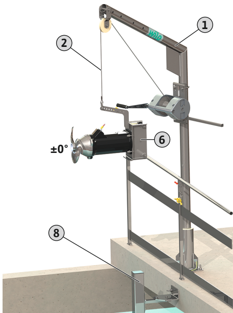
Fig. 6: Περιστροφή αναδευτήρα επάνω από τη λεκάνη
