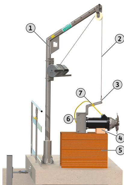
Fig. 5: Προετοιμασία αναδευτήρα
