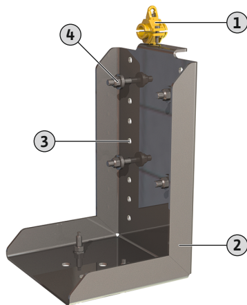
Fig. 16: Υποστήριγμα στερέωσης για επιδαπέδια εγκατάσταση
