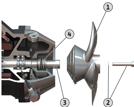
Fig. 13: Αντικατάσταση έλικα
