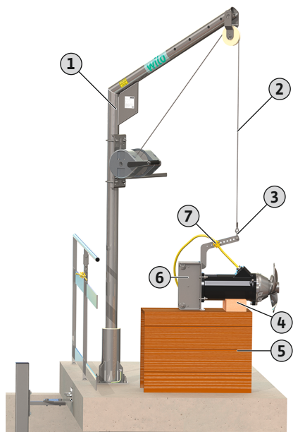
Fig. 5: Příprava míchadla
