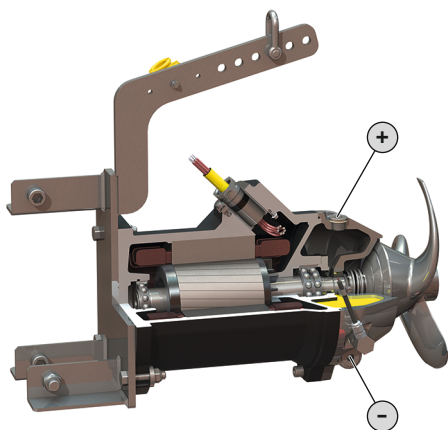
Fig. 12: Výměna oleje
