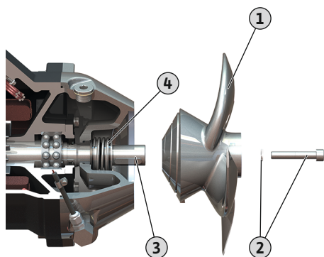
Fig. 13: Výměna vrtule
