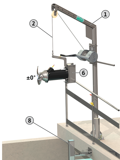
Fig. 6: Natočte míchadlo nad jímku
