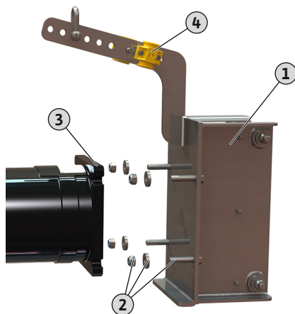
Fig. 15: Výměna rámu
