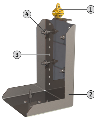
Fig. 16: Konzola pro montáž na podlahu
