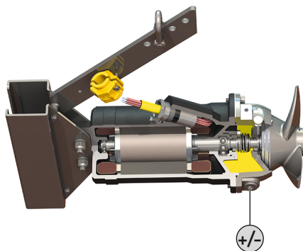
Fig. 11: Výměna oleje
