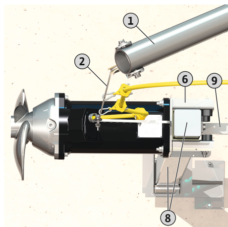
Fig. 7: A keverőmű a leeresztő szerkezeten
