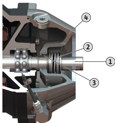
Fig. 14: A csúszógyűrűs tömítés cseréje
