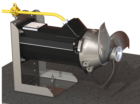
Fig. 4: Talajra szerelhető változat
