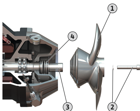
Fig. 13: A propeller cseréje
