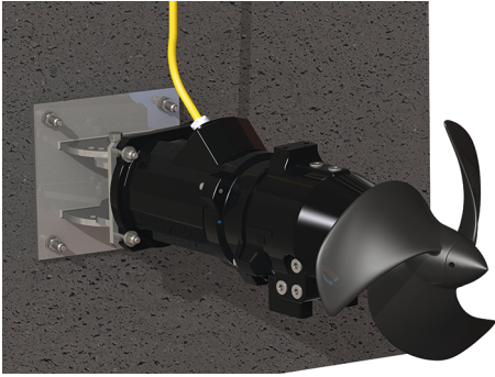
Fig. 3: Zidna montaža
