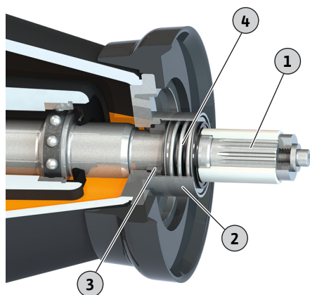
Fig. 14: Zamena mehaničkog zaptivača
