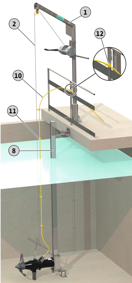
Fig. 8: Mehanizam za mešanje postavljen u graničnom položaju
