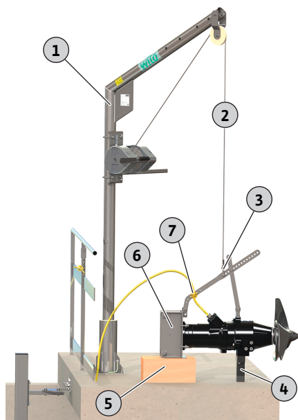
Fig. 5: Priprema mehanizma za mešanje
