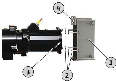
Fig. 16: Zameniti okvir
