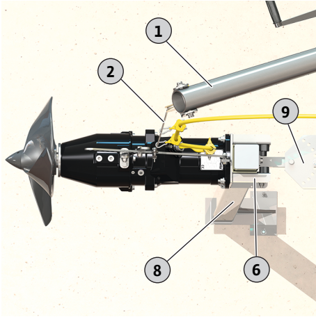
Fig. 7: Mehanizam za mešanje na napravi za spuštanje
