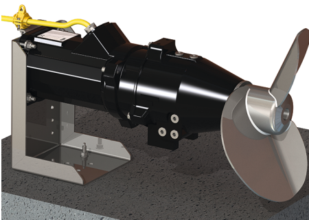
Fig. 4: Montaža na pod
