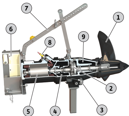
Fig. 2: Pregled mehanizma za mešanje sa uronjivim motorom
