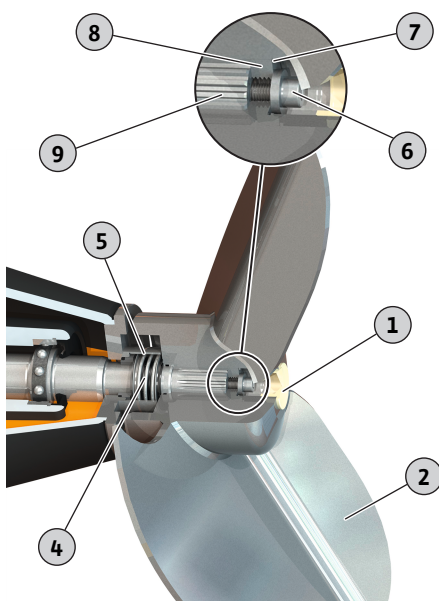
Fig. 13: Zamena propelera (nerđajući čelik)
