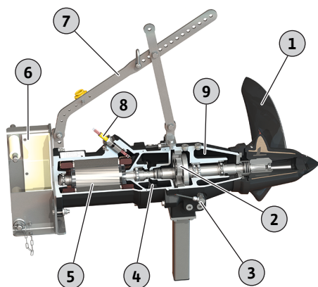
Fig. 2: Обзор погружная мешалка
