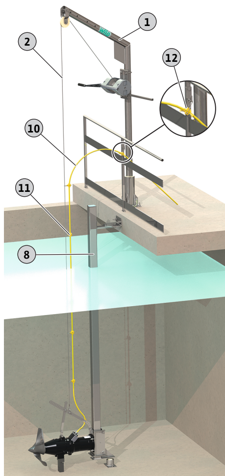
Fig. 8: Мешалка поставлена на жесткий упор
