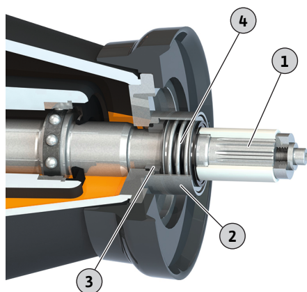
Fig. 14: Замена торцевого уплотнения
