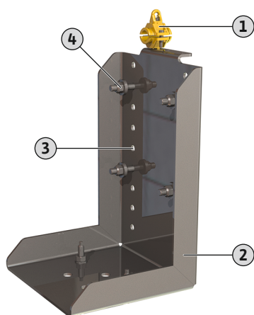
Fig. 17: Консоль для напольного монтажа
