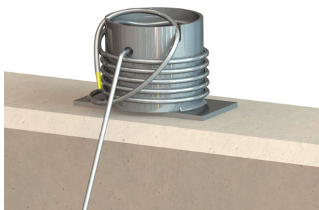
Fig. 9: Подъемное устройство закреплено на швартовой тумбе
