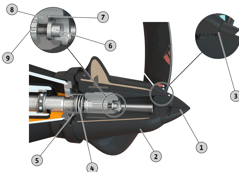
Fig. 12: Замена пропеллера (пластик)
