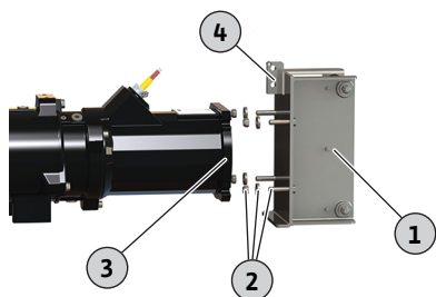
Fig. 16: Замена рамы
