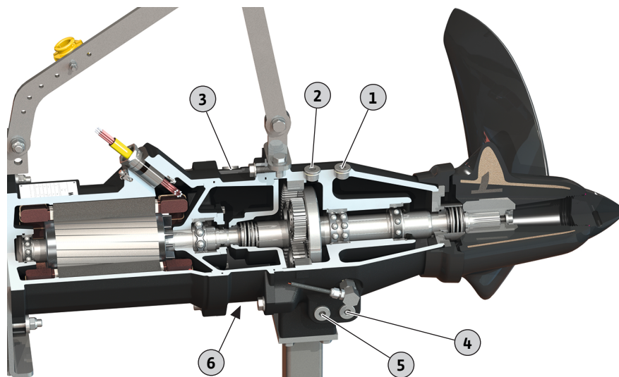
Fig. 11: Замена масла
