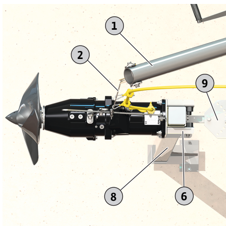
Fig. 7: Мешалка у погружного устройства
