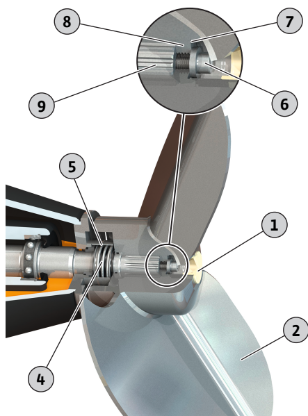
Fig. 13: Замена пропеллера (нержавеющая сталь)
