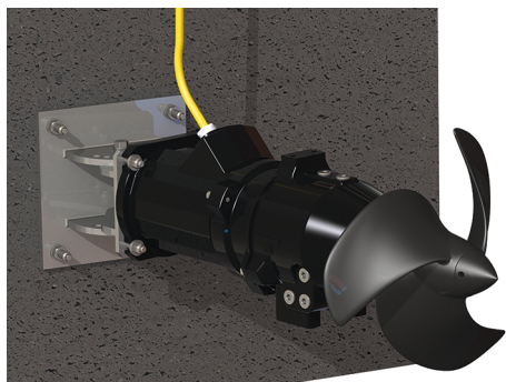
Fig. 3: Настенный монтаж
