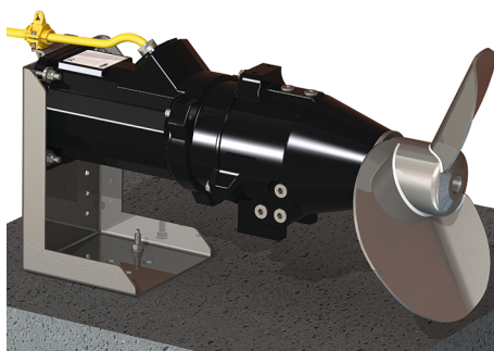
Fig. 4: Напольный монтаж
