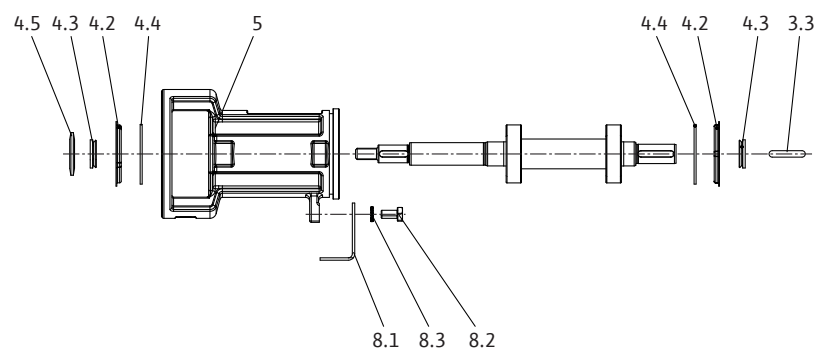
Fig. 26: Suport lagăr
