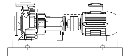
Fig. 5: Amplasarea pe fundație a agregatului
