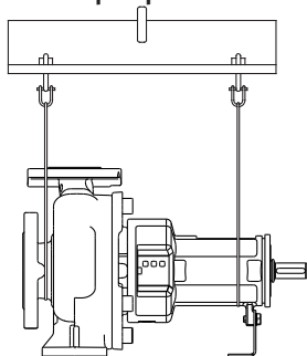
Fig. 3: Fixarea pompei
