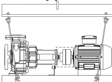
Fig. 4: Fixarea agregatului
