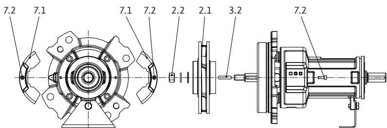
Fig. 20: Demontarea unității de împingere
