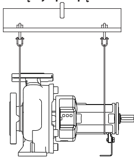
Fig. 3: Podłączyć pompę
