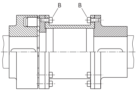
Fig. 18: Śruba mocująca B połówek sprzęgła
