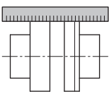
Fig. 14: Kontrola osiowania promieniowego przy wykorzystaniu liniatu
