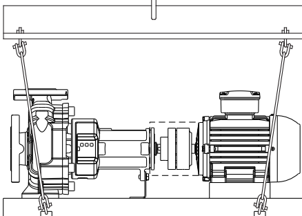
Fig. 4: Podłączyć urządzenie
