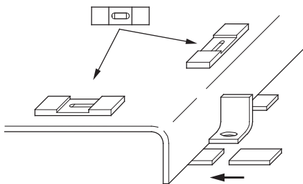
Fig. 8: Niwelowanie i wyrównywanie płyty podstawy
