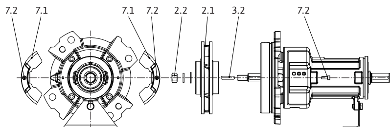
Fig. 29: Zamontować jednostkę wsuwaną
